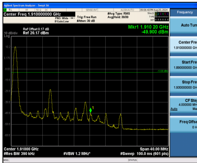
Band2-20MHz-16QAM-19100-27RB#0
