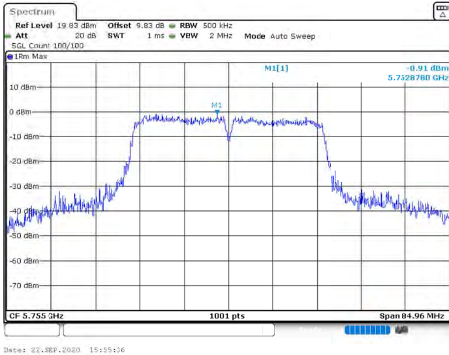
PSD NVNT 802.11n(HT40) 5755MHz Ant1
