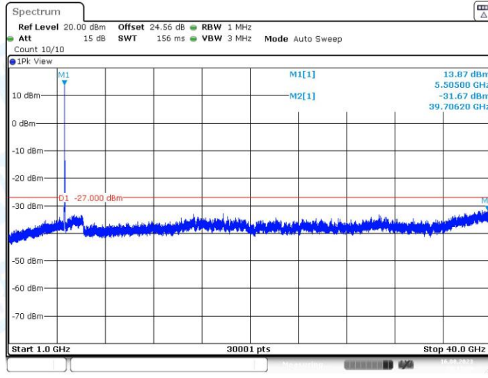
11A_Ant1_5500_1000~40000
