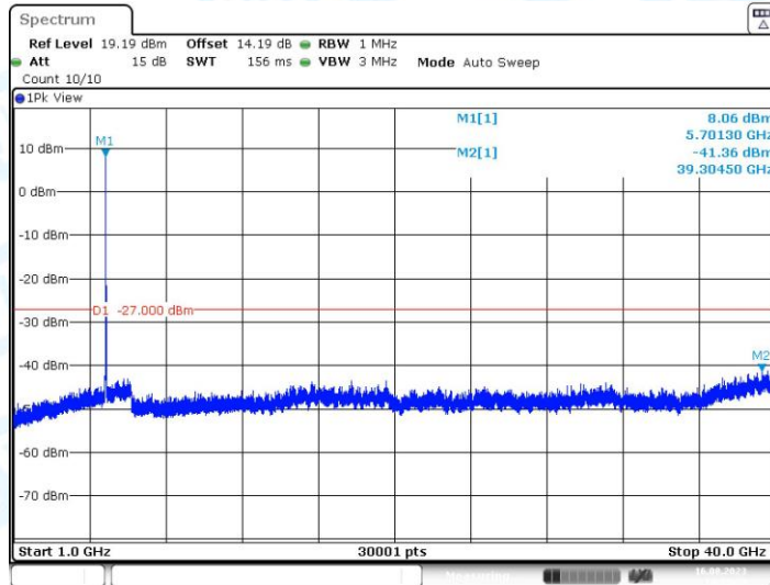
11N20MIMO_Ant1_5700_1000~40000
