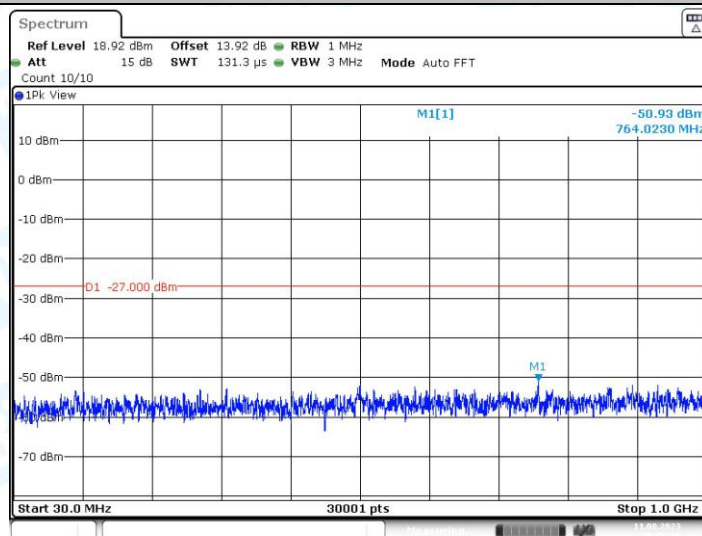
11N20MIMO_Ant1_5785_30~1000
