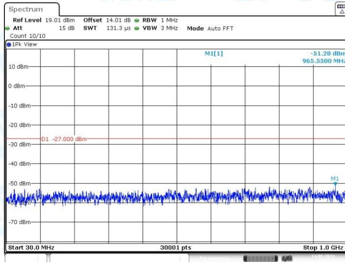
11N40MIMO_Ant2_5795_30~1000
