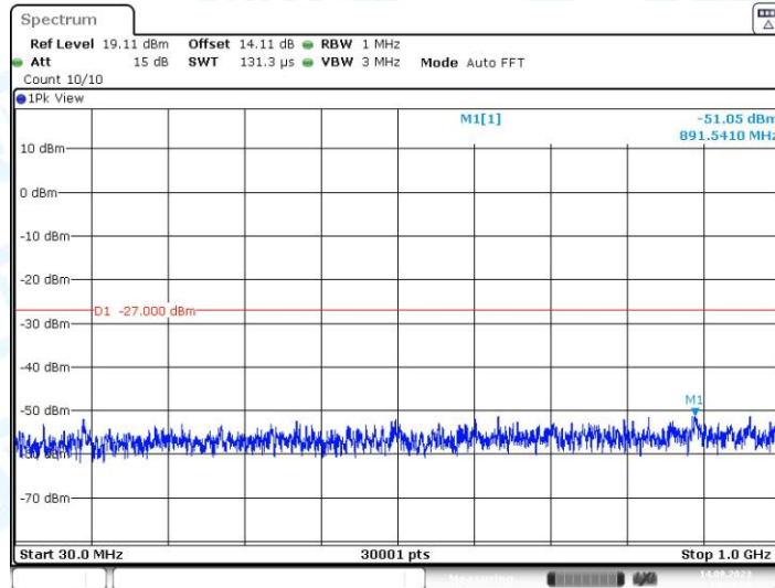
11N40MIMO_Ant2_5755_30~1000
