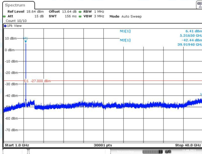
11N20MIMO_Ant1_5320_1000~40000
