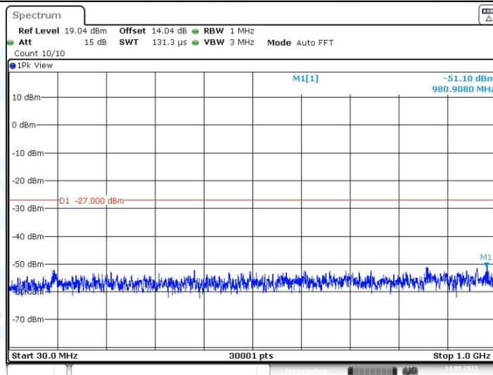
11N40MIMO_Ant2_5550_30~1000
