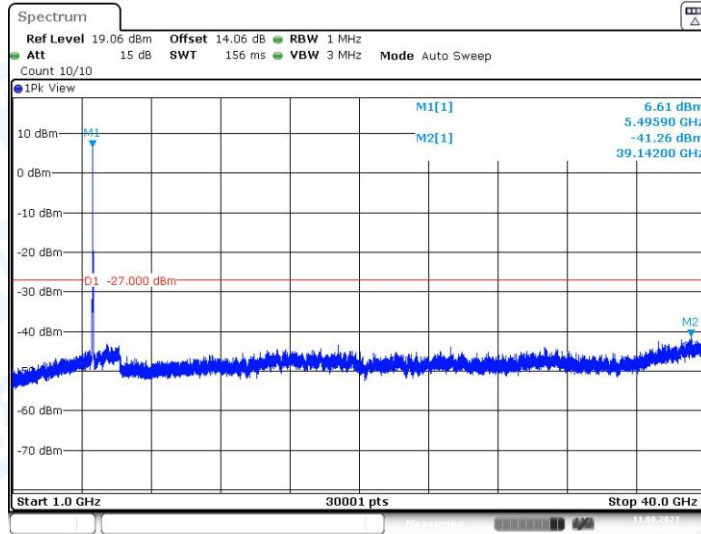
11N20MIMO_Ant1_5500_1000~40000
