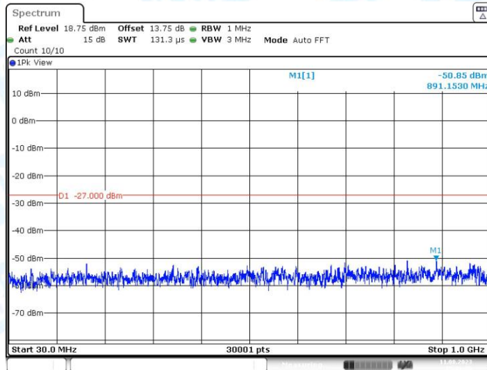
11N20MIMO_Ant2_5320_30~1000
