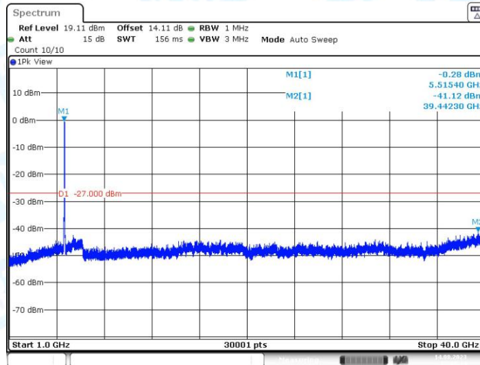
11N40MIMO_Ant2_5510_1000~40000
