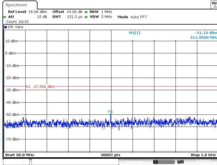
11N20MIMO_Ant1_5500_30~1000
