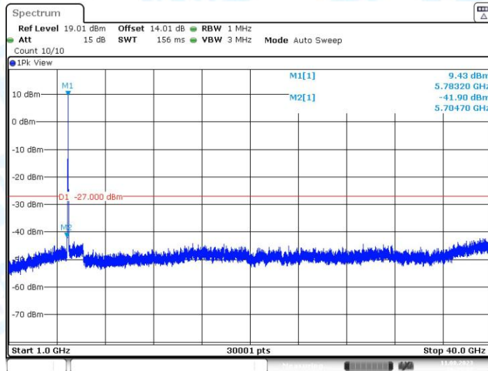
11N20MIMO_Ant2_5785_1000~40000
