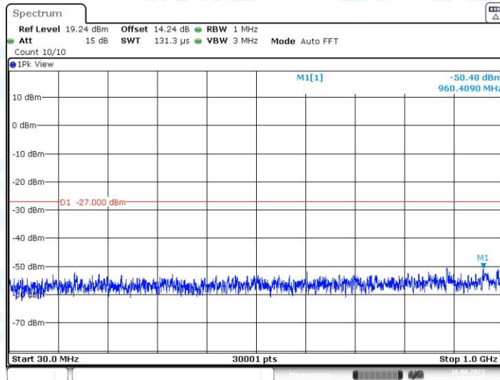
11N20MIMO_Ant2_5700_30~1000
