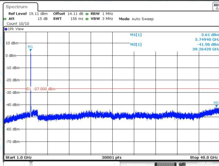
11N40MIMO_Ant2_5755_1000~40000
