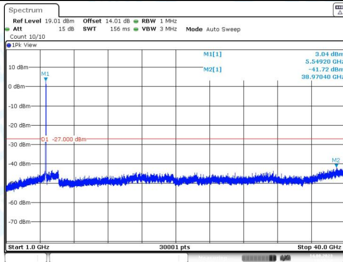
11N40MIMO_Ant1_5550_1000~40000
