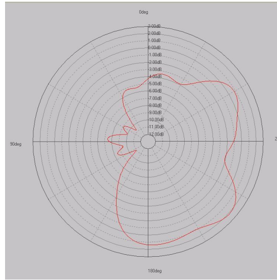
E2 plane
