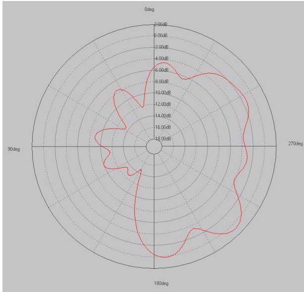
E1 plane
