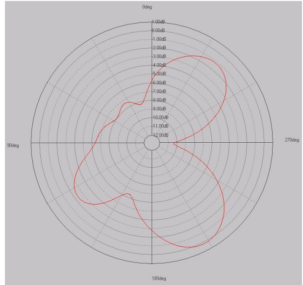
E2 plane
