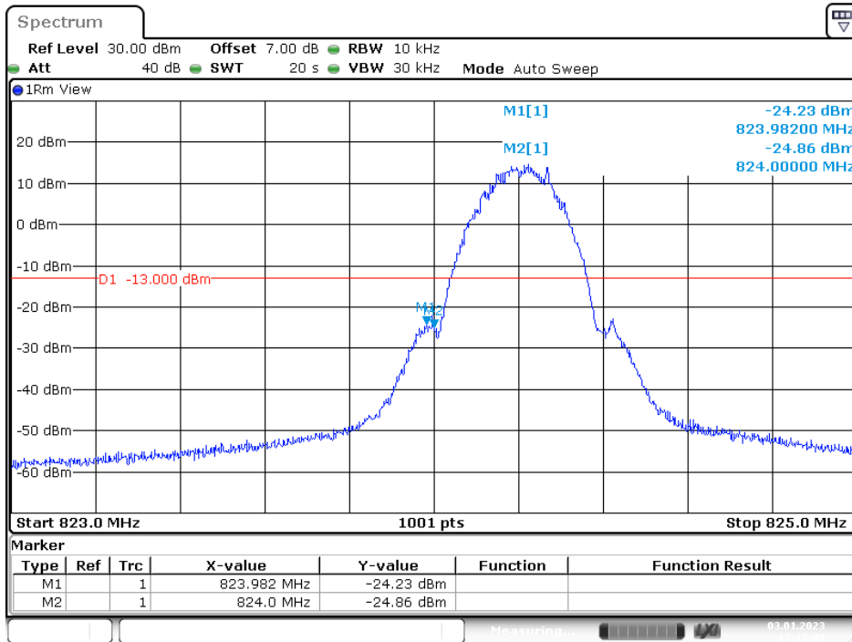
Left Band Edge for GSM (GMSK) Mode
