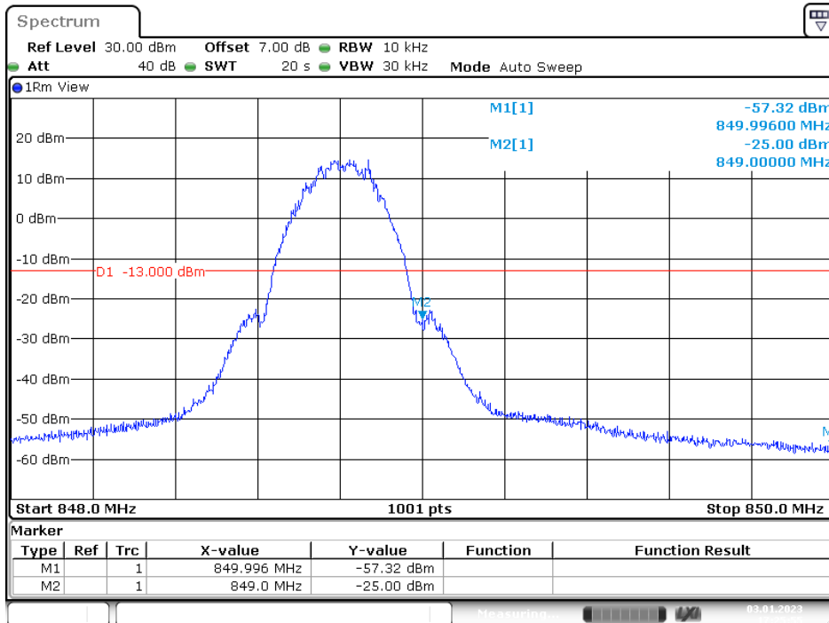
Right Band Edge for GSM (GMSK) Mode
