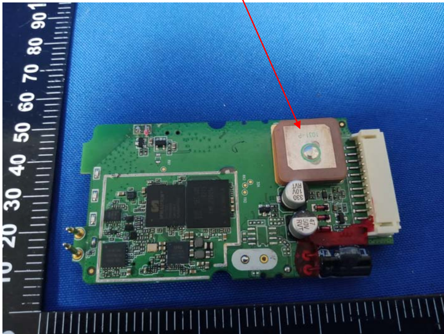
GPS ANT
