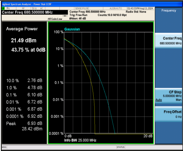
Band71-10MHz-QPSK-133297-1RB#0-PASS
