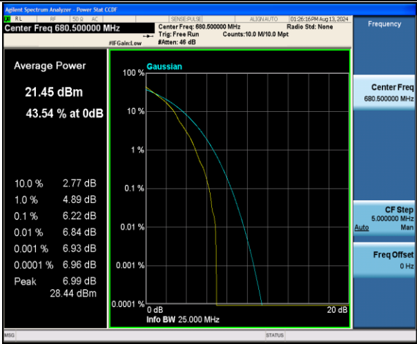
Band71-5MHz-QPSK-133297-1RB#0-PASS
