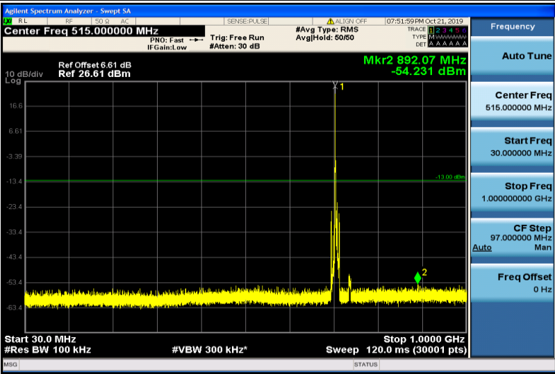
Band12-5MHz-QPSK-23155-1RB#0-30~1000MHz
