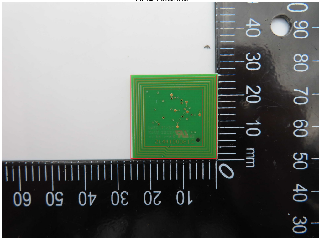
RFID Antenna
