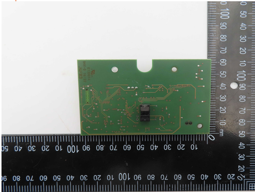
RFID Antenna
