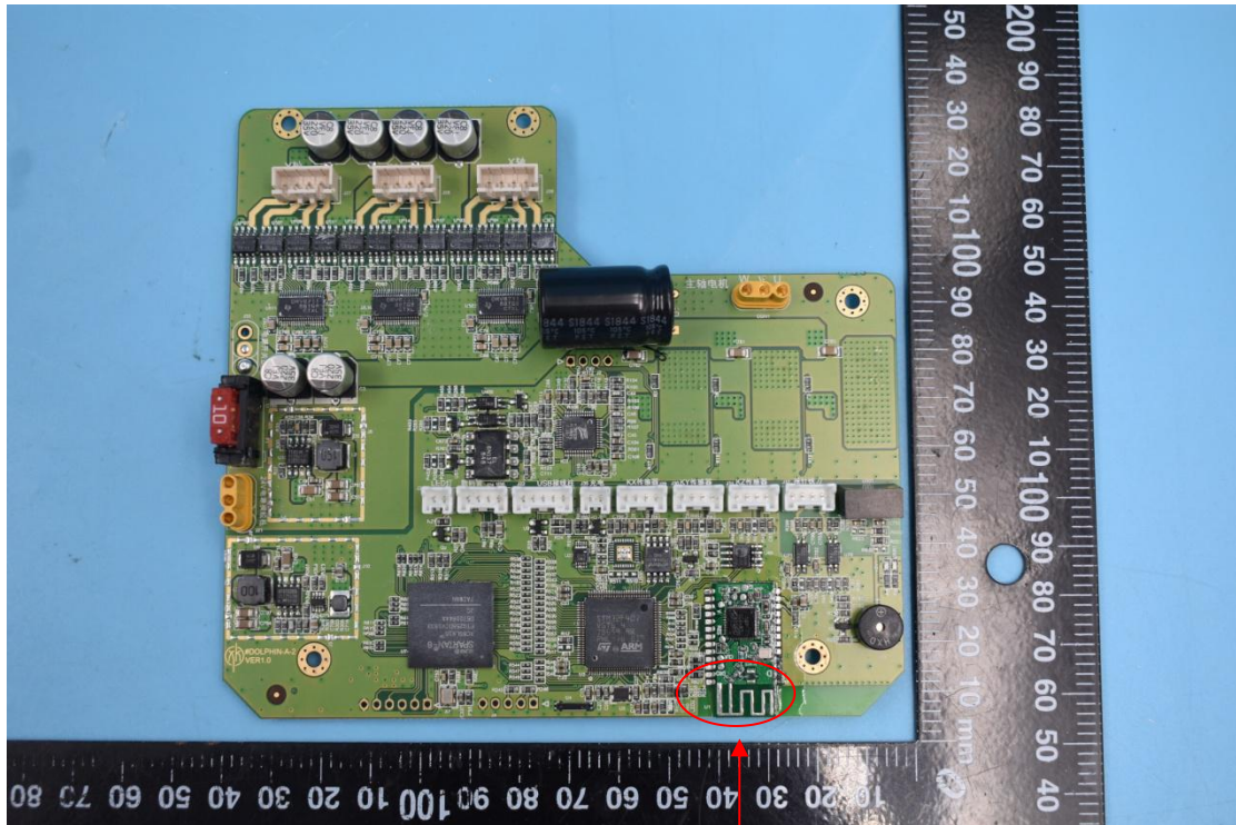
BLE Antenna
