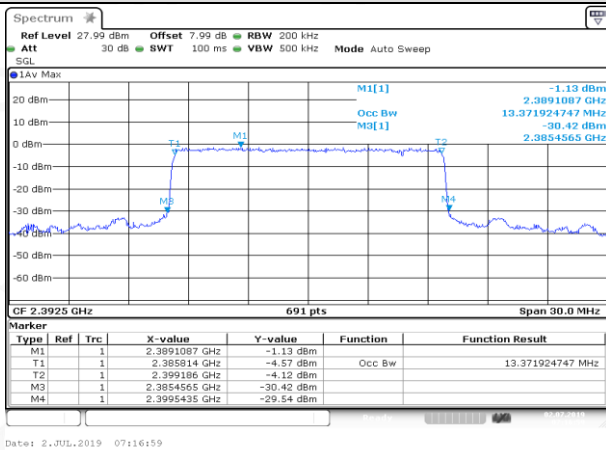
HCH_QPSK_75RB#0
