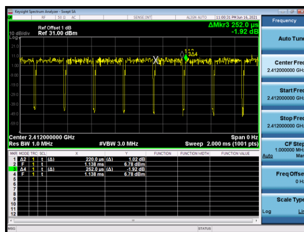
Mode 2 2412MHz
