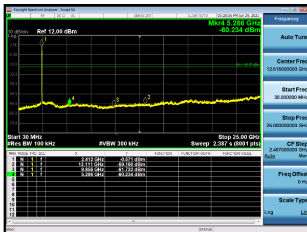
Mode 5 2412MHz
