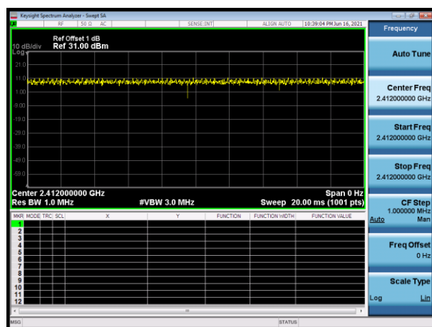
Mode 3 2412MHz
