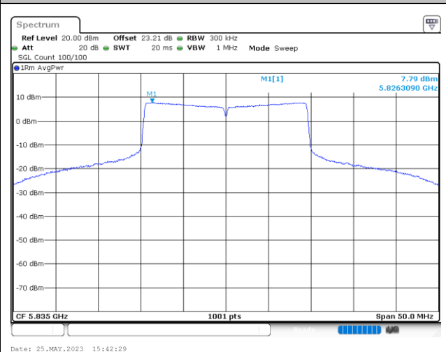
MIMO Ant. 2
