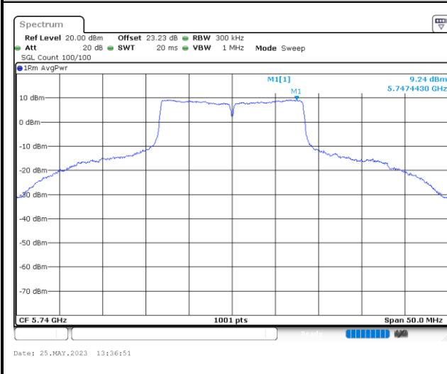
MIMO Ant. 0
