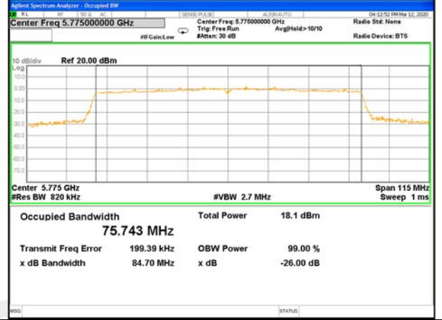
W58_11ac80_26BW_99%_Bandwidth_5775M
