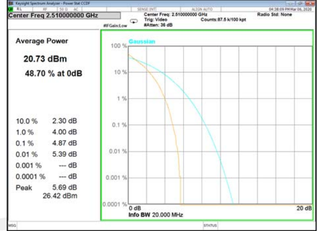
B7_100_Q16_Lower
