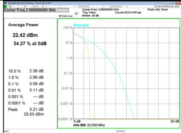
B7_1_Q16_High
