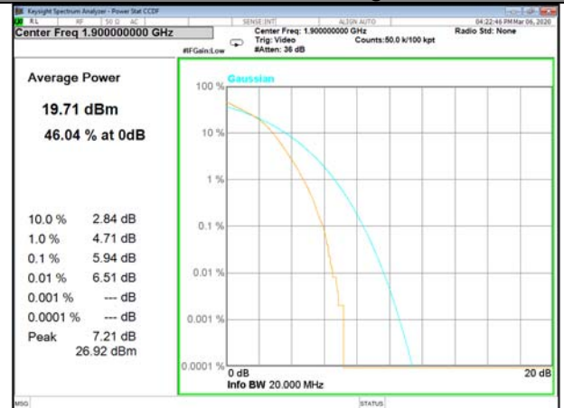
B2_100_Q16_High
