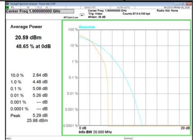
B2_1_Q16_High
