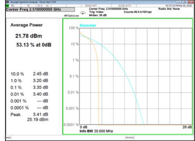
B7_1_Q16_Lower
