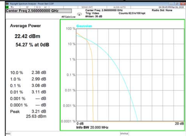
B7_1_Q16_High
