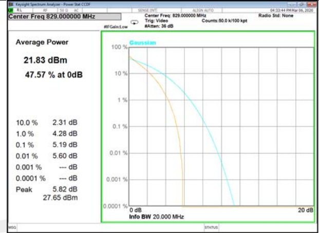
B5_50_Q16_Lower
