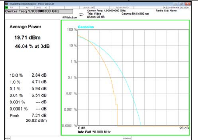
B2_100_Q16_High
