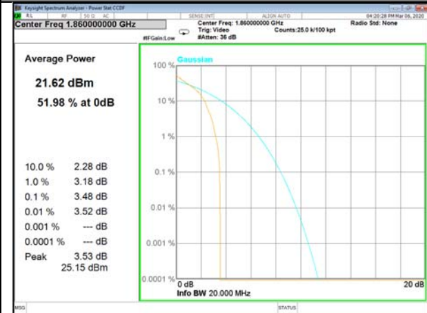
B2_1_Q16_Lower
