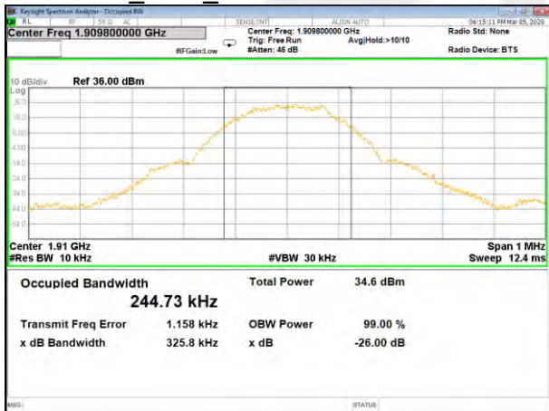
GSM_1900_Higher_26BW_and_99%
