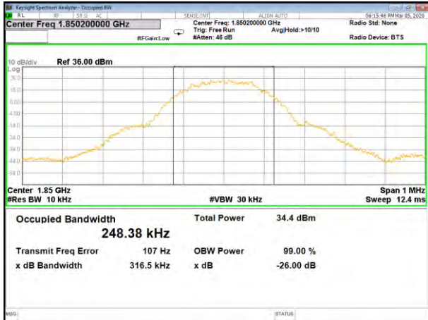
GSM_1900_Lower_26BW_and_99%
