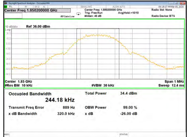
GPRS_1900_Lower_26BW_and_99%
