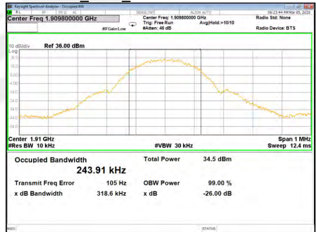
GPRS_1900_Higher_26BW_and_99%
