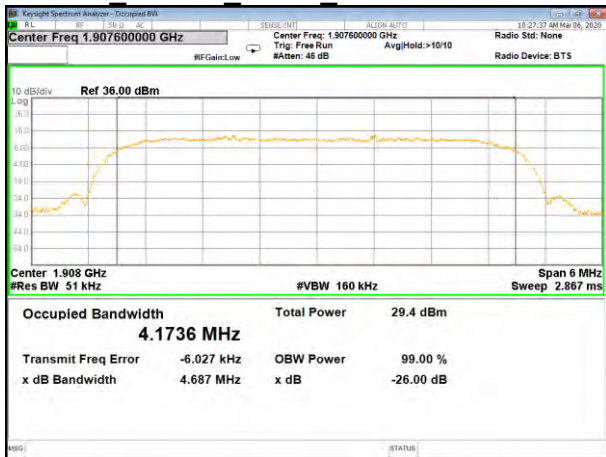
B2_HSUPA_Higher_26BW and 99%
