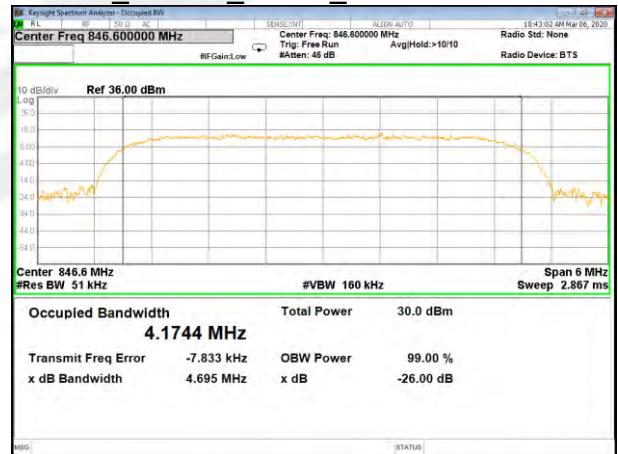
B5_HSDPA_Higher_26BW and 99%
