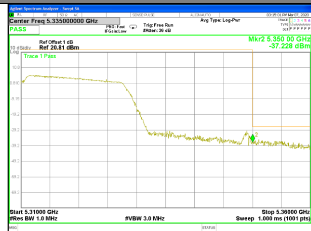
W53_11ac40_Higher_Band edge
