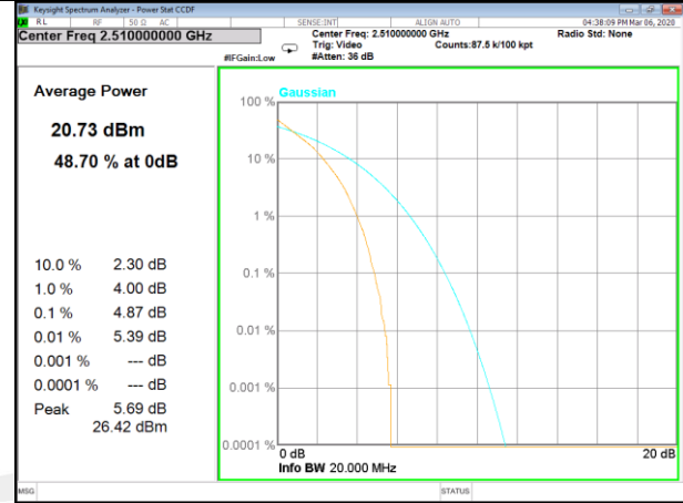
B7_100_Q16_Lower
