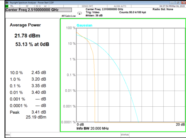
B7_1_Q16_Lower
