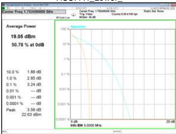
HSPA4_Higher_
