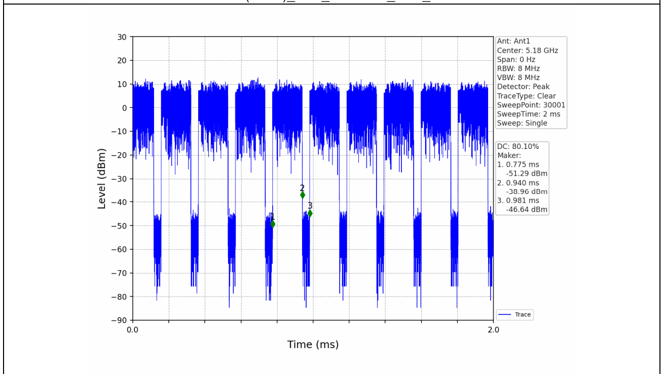
802.11n(HT20)_LCH_5180MHz_Ant1_NTNV
