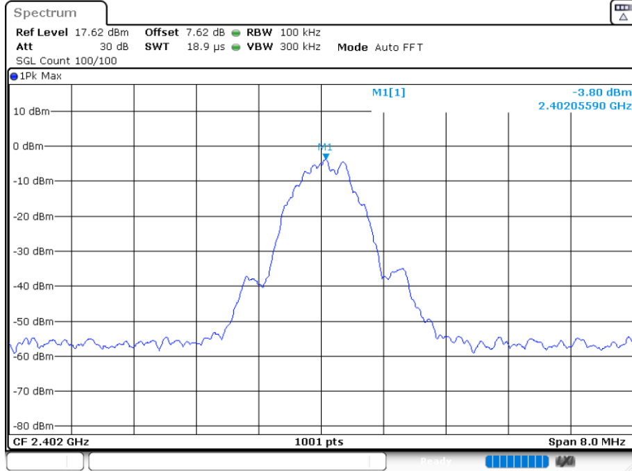
Band Edge NVNT BLE-1M 2402MHz Ref
