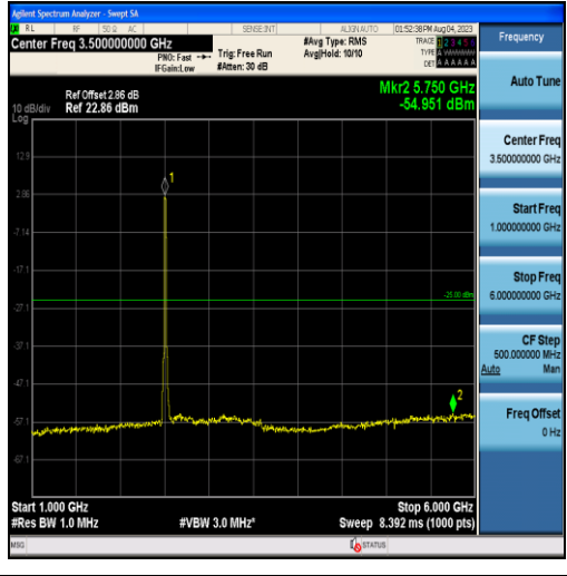
Band41-20MHz-QPSK-39750-100RB#0-Range2:1000~6000MHz
