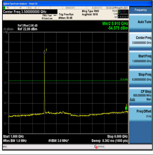
Band41-10MHz-16QAM-39700-50RB#0-Range2:1000~6000MHz
