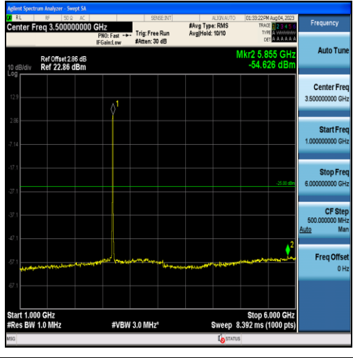
Band41-10MHz-QPSK-41540-50RB#0-Range2:1000~6000MHz
