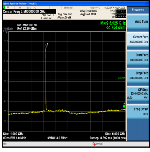
Band41-10MHz-QPSK-40620-50RB#0-Range2:1000~6000MHz
