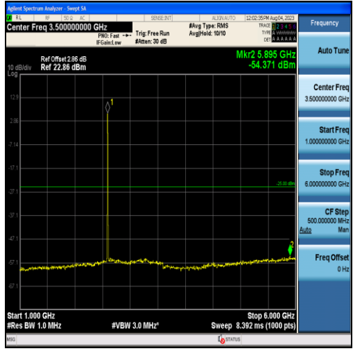
Band41-5MHz-16QAM-40620-25RB#0-Range2:1000~6000MHz
