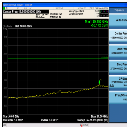
Band41-20MHz-QPSK-41490-100RB#0-Range3:6000~27000MHz
