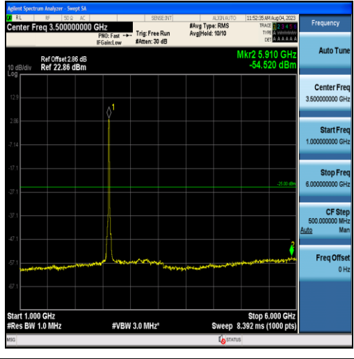
Band38-20MHz-QPSK-38150-100RB#0-Range2:1000~6000MHz
