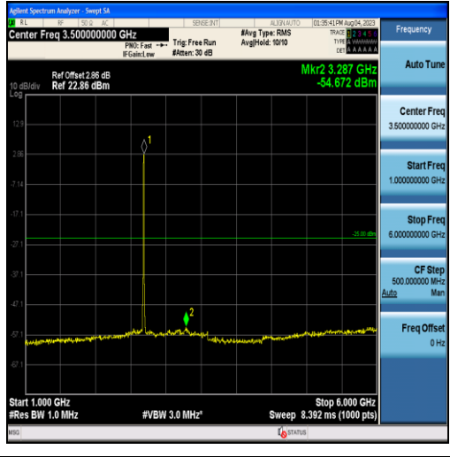
Band41-10MHz-16QAM-41540-50RB#0-Range2:1000~6000MHz
