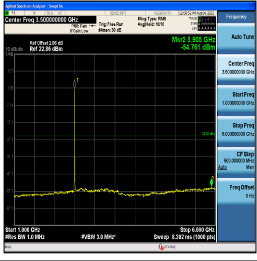
Band41-5MHz-QPSK-39675-25RB#0-Range2:1000~6000MHz
