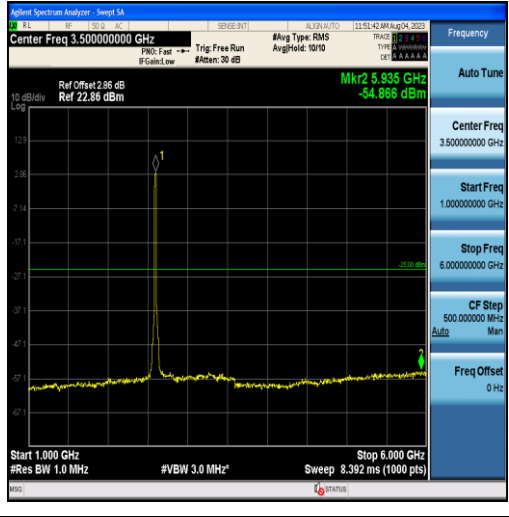
Band38-20MHz-QPSK-38000-100RB#0-Range2:1000~6000MHz
