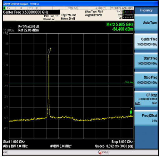
Band41-20MHz-QPSK-40620-100RB#0-Range2:1000~6000MHz
