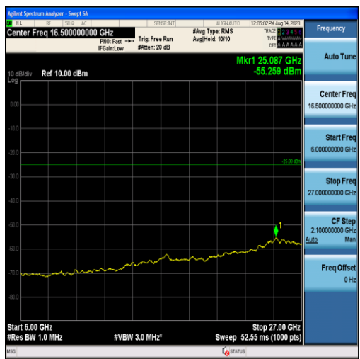
Band41-5MHz-16QAM-40620-25RB#0-Range3:6000~27000MHz
