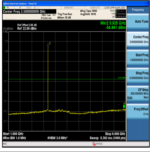
Band41-5MHz-QPSK-41565-25RB#0-Range2:1000~6000MHz
