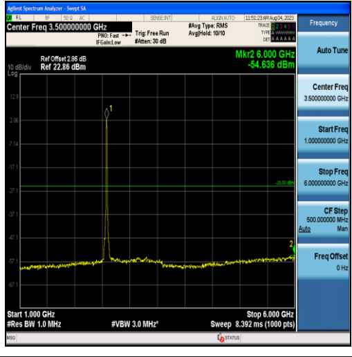
Band38-20MHz-16QAM-37850-100RB#0-Range2:1000~6000MHz
