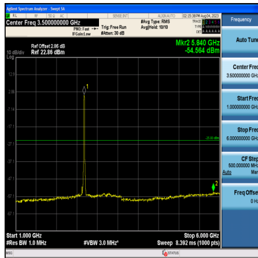
Band41-20MHz-QPSK-41490-100RB#0-Range2:1000~6000MHz
