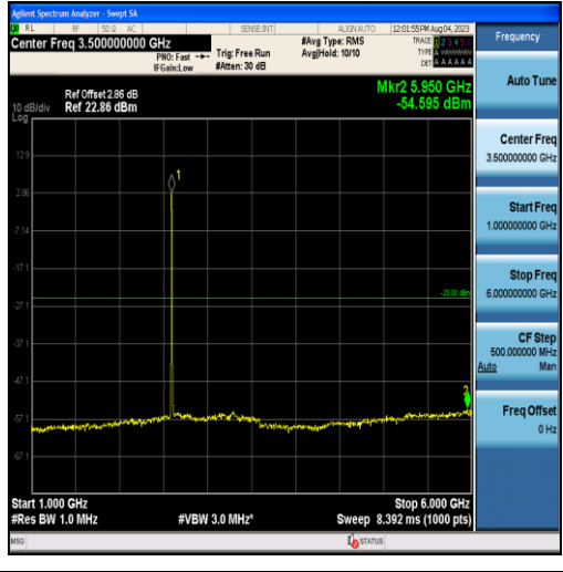
Band41-5MHz-QPSK-40620-25RB#0-Range2:1000~6000MHz
