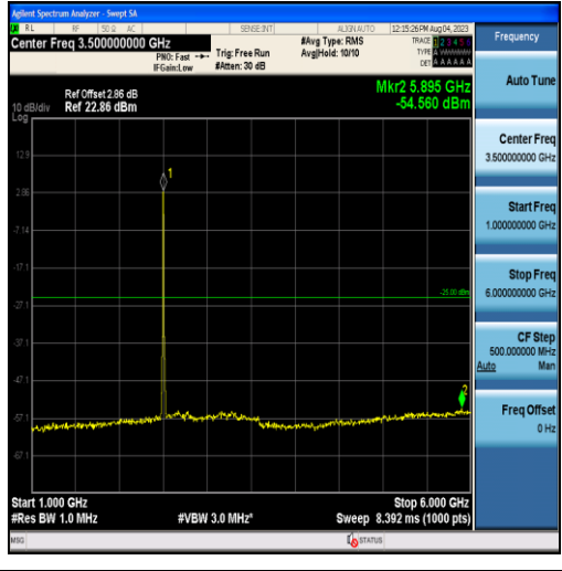
Band41-10MHz-QPSK-39700-50RB#0-Range2:1000~6000MHz
