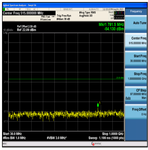
Band41-10MHz-QPSK-39700-50RB#0-Range1:30~1000MHz
