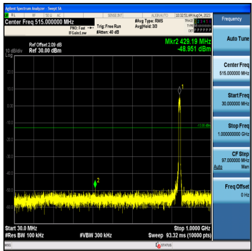
Band26-10MHz-QPSK-26990-50RB#0-Range1:30~1000MHz
