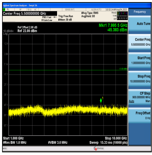
Band26-10MHz-QPSK-26840-50RB#0-Range2:1000~10000MHz
