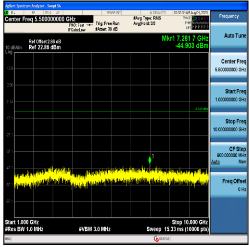
Band26-10MHz-QPSK-26915-50RB#0-Range2:1000~10000MHz
