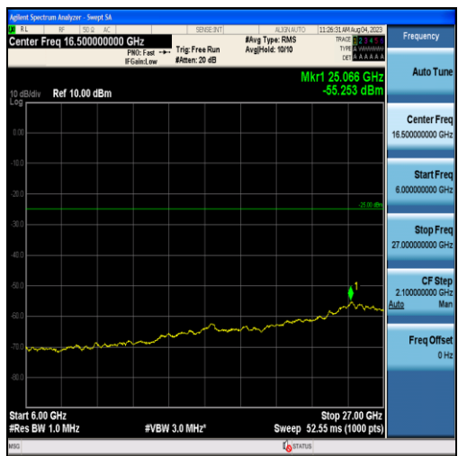
Band38-10MHz-QPSK-38000-50RB#0-Range3:6000~27000MHz
