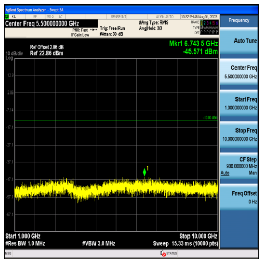
Band26-10MHz-QPSK-26990-50RB#0-Range2:1000~10000MHz
