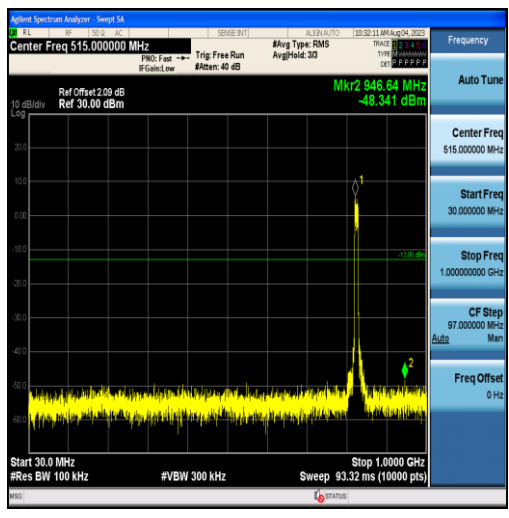
Band26-10MHz-QPSK-26840-50RB#0-Range1:30~1000MHz
