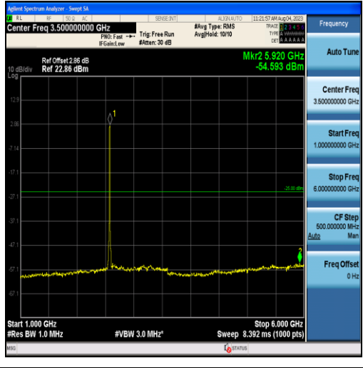
Band38-10MHz-QPSK-37800-50RB#0-Range2:1000~6000MHz
