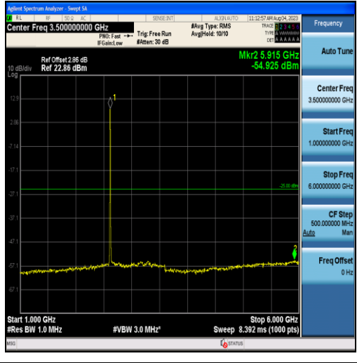
Band38-5MHz-QPSK-38225-25RB#0-Range2:1000~6000MHz
