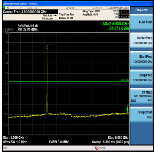
Band38-10MHz-QPSK-38000-50RB#0-Range2:1000~6000MHz
