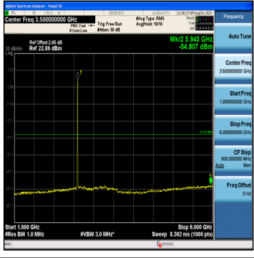
Band38-5MHz-QPSK-38000-25RB#0-Range2:1000~6000MHz
