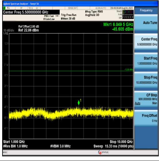
Band26-3MHz-QPSK-26775-15RB#0-Range2:1000~10000MHz
