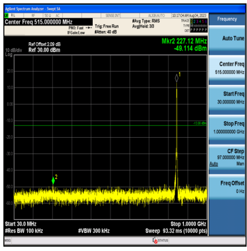
Band26-3MHz-QPSK-27025-15RB#0-Range1:30~1000MHz
