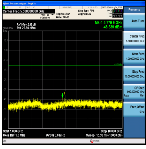
Band26-5MHz-QPSK-26765-25RB#0-Range2:1000~10000MHz
