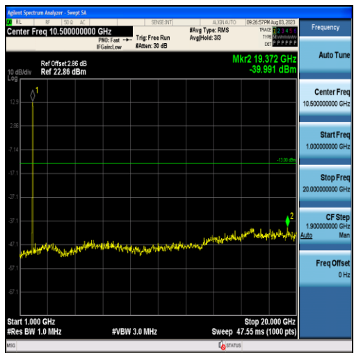
Band25-20MHz-QPSK-26365-100RB#0-Range2:1000~20000MHz
