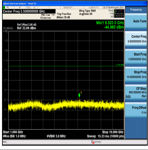
Band26-3MHz-QPSK-27025-15RB#0-Range2:1000~10000MHz
