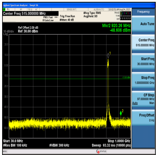
Band26-10MHz-QPSK-26740-50RB#0-Range1:30~1000MHz
