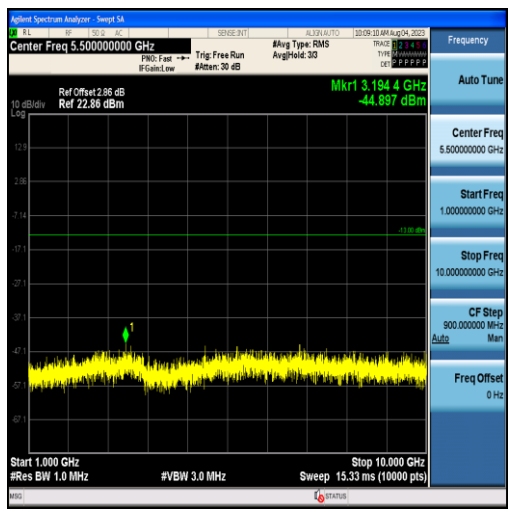
Band26-1.4MHz-QPSK-26797-6RB#0-Range2:1000~10000MHz
