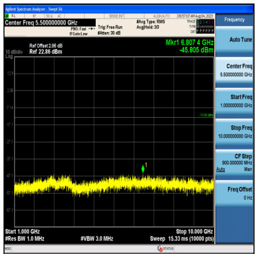
Band26-5MHz-QPSK-26740-25RB#0-Range2:1000~10000MHz
