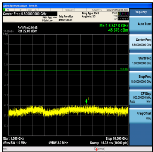
Band26-10MHz-QPSK-26740-50RB#0-Range2:1000~10000MHz
