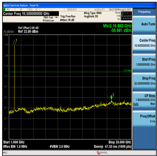
Band25-20MHz-16QAM-26365-100RB#0-Range2:1000~20000MHz
