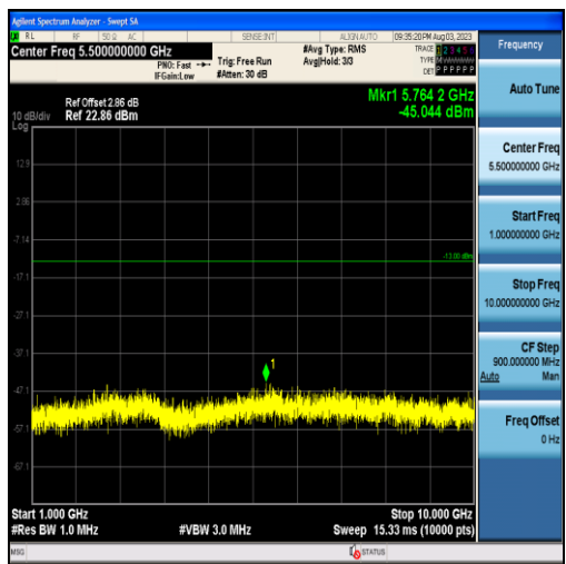
Band26-1.4MHz-QPSK-26697-6RB#0-Range2:1000~10000MHz
