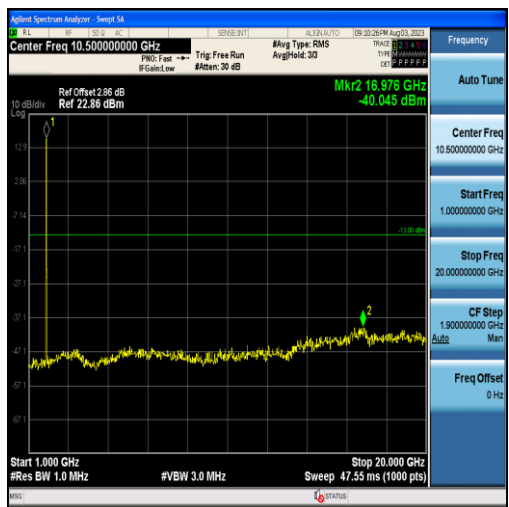
Band25-10MHz-QPSK-26090-50RB#0-Range2:1000~20000MHz
