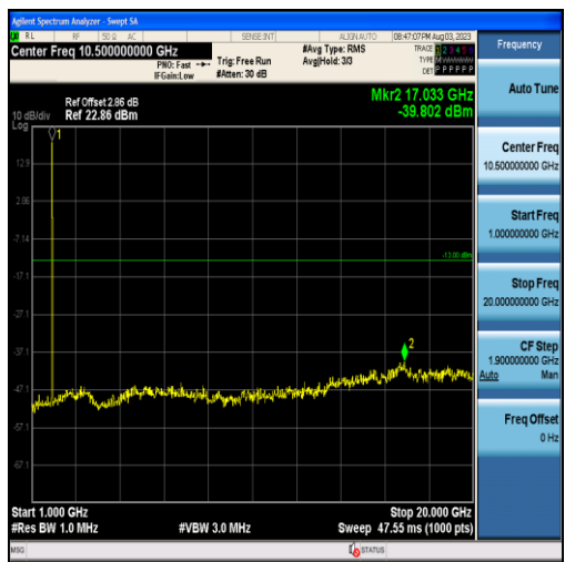
Band25-1.4MHz-16QAM-26365-6RB#0-Range2:1000~20000MHz
