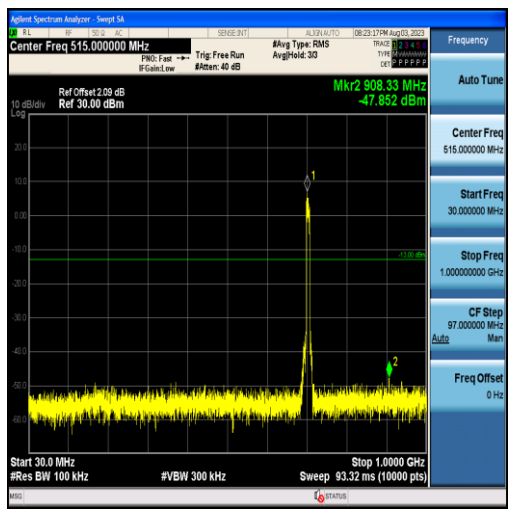
Band12-10MHz-QPSK-23130-50RB#0-Range1:30~1000MHz
