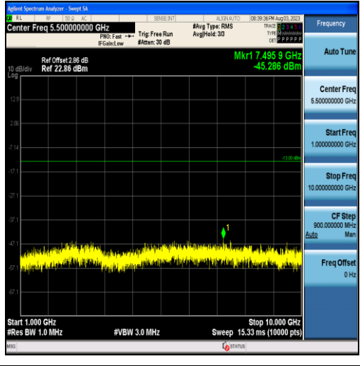
Band13-10MHz-QPSK-23230-50RB#0-Range2:1000~10000MHz
