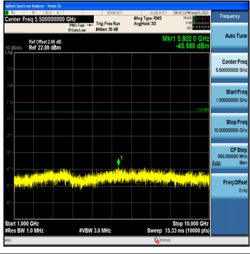
Band13-5MHz-QPSK-23205-25RB#0-Range2:1000~10000MHz
