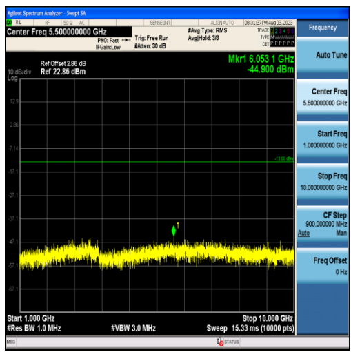
Band13-5MHz-QPSK-23230-25RB#0-Range2:1000~10000MHz
