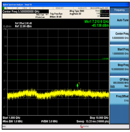
Band12-10MHz-QPSK-23130-50RB#0-Range2:1000~10000MHz
