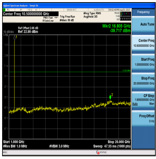
Band25-5MHz-QPSK-26365-25RB#0-Range2:1000~20000MHz
