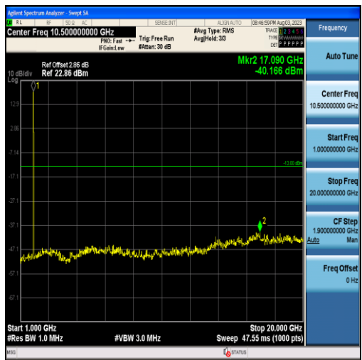
Band25-1.4MHz-QPSK-26365-6RB#0-Range2:1000~20000MHz
