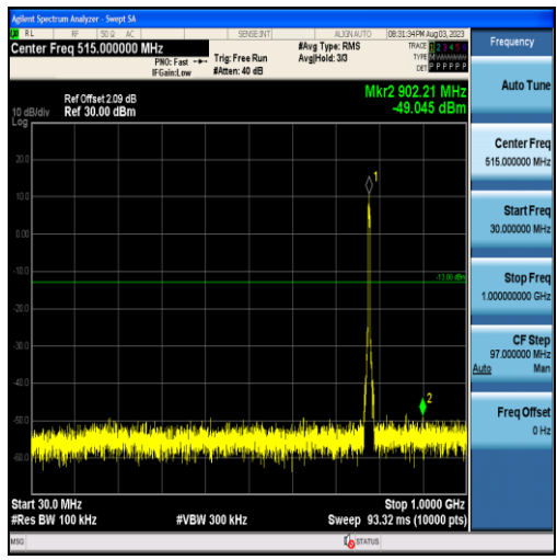
Band13-5MHz-QPSK-23230-25RB#0-Range1:30~1000MHz
