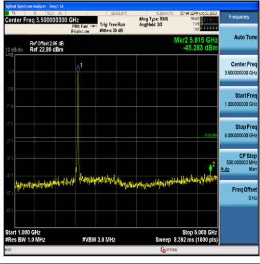
Band7-20MHz-16QAM-21350-100RB#0-Range2:1000~6000MHz
