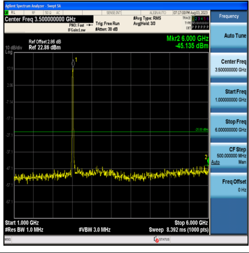
Band7-20MHz-QPSK-20850-100RB#0-Range2:1000~6000MHz
