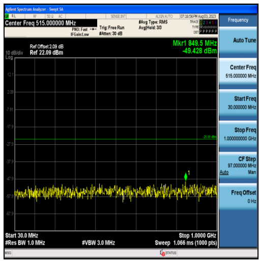
Band7-20MHz-QPSK-20850-100RB#0-Range1:30~1000MHz
