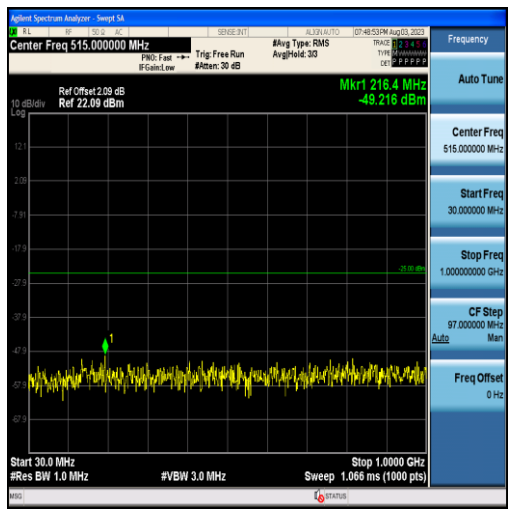
Band7-20MHz-QPSK-21350-100RB#0-Range1:30~1000MHz
