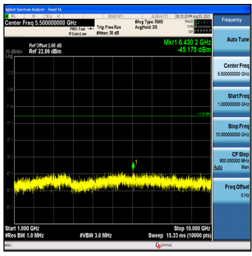
Band12-5MHz-QPSK-23095-25RB#0-Range2:1000~10000MHz
