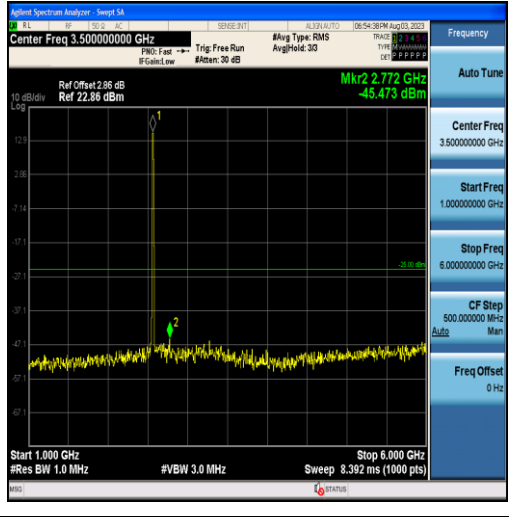
Band7-10MHz-16QAM-21400-50RB#0-Range2:1000~6000MHz
