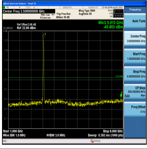
Band7-20MHz-QPSK-21100-100RB#0-Range2:1000~6000MHz
