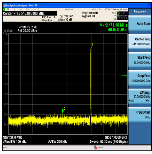
Band12-1.4MHz-QPSK-23017-6RB#0-Range 1:30~1000MHz
