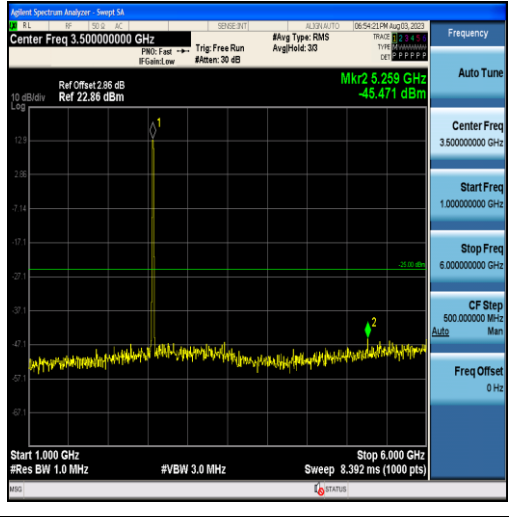
Band7-10MHz-QPSK-21400-50RB#0-Range2:1000~6000MHz
