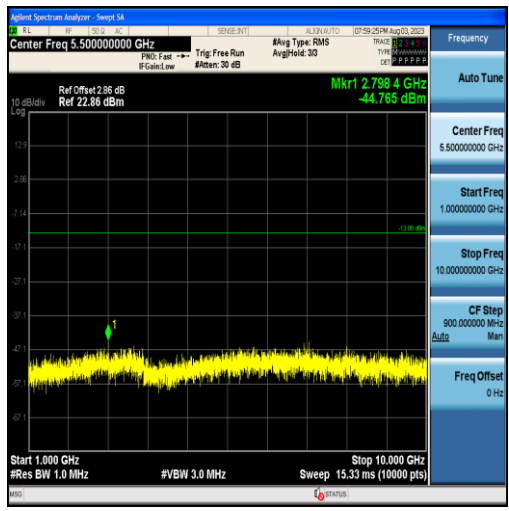
Band12-1.4MHz-QPSK-23017-6RB#0-Range2:1000~10000MHz
