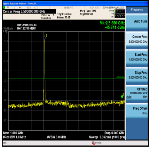
Band7-20MHz-QPSK-21350-100RB#0-Range2:1000~6000MHz
