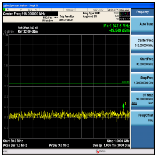
Band7-10MHz-QPSK-21400-50RB#0-Range1:30~1000MHz
