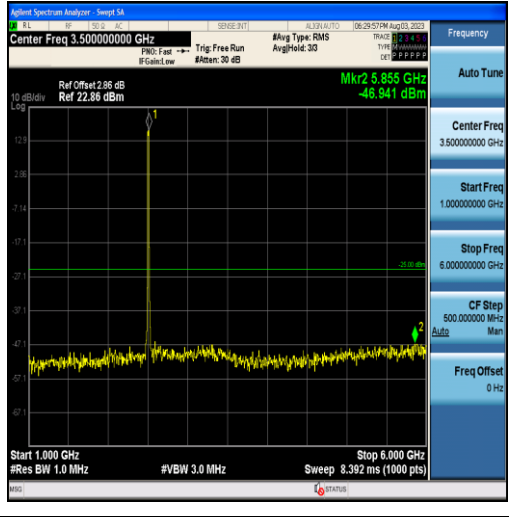
Band7-10MHz-QPSK-20800-50RB#0-Range2:1000~6000MHz
