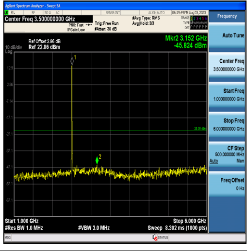
Band7-5MHz-QPSK-20775-25RB#0-Range2:1000~6000MHz
