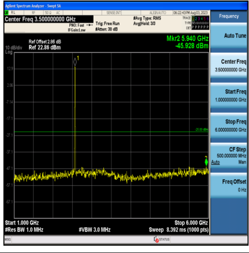
Band7-5MHz-QPSK-21425-25RB#0-Range2:1000~6000MHz
