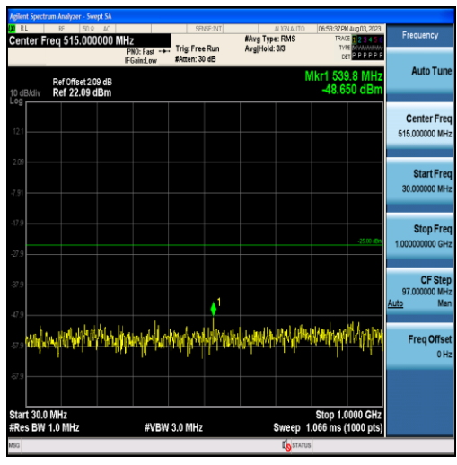
Band7-10MHz-QPSK-21100-50RB#0-Range1:30~1000MHz
