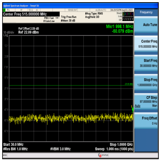
Band7-10MHz-QPSK-20800-50RB#0-Range1:30~1000MHz
