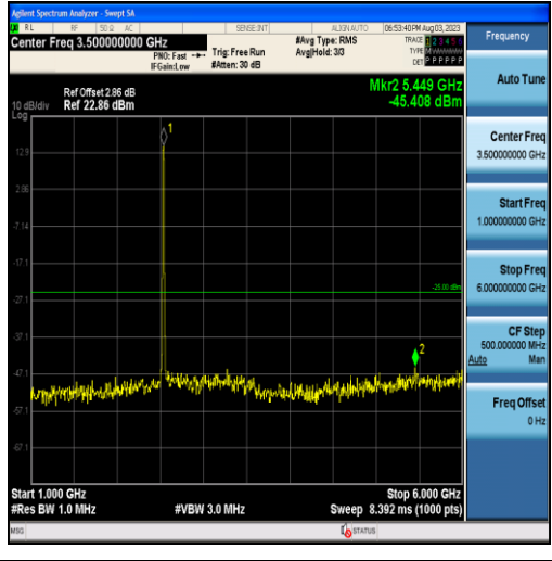
Band7-10MHz-QPSK-21100-50RB#0-Range2:1000~6000MHz
