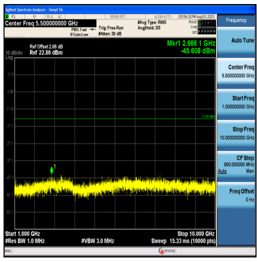
Band5-3MHz-QPSK-20525-15RB#0-Range2:1000~10000MHz
