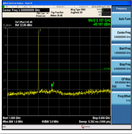
Band7-10MHz-16QAM-20800-50RB#0-Range2:1000~6000MHz
