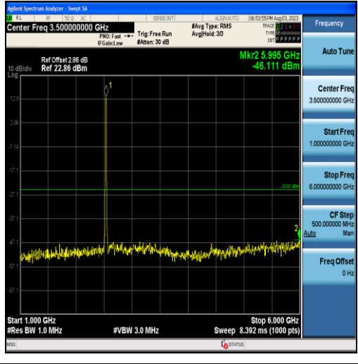
Band7-10MHz-16QAM-21100-50RB#0-Range2:1000~6000MHz
