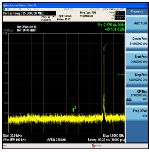
Band5-3MHz-QPSK-20415-15RB#0-Range1:30~1000MHz
