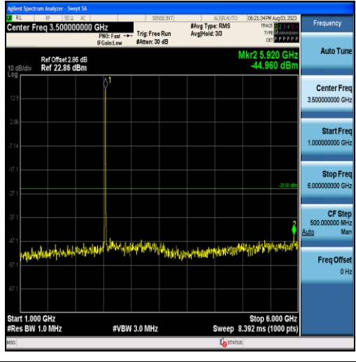
Band7-5MHz-QPSK-21100-25RB#0-Range2:1000~6000MHz
