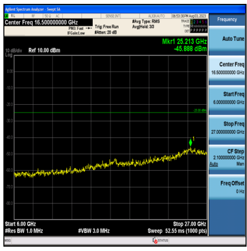
Band7-10MHz-16QAM-20800-50RB#0-Range3:6000~27000MHz
