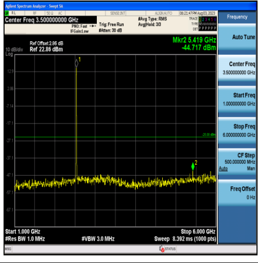
Band7-5MHz-16QAM-21100-25RB#0-Range2:1000~6000MHz
