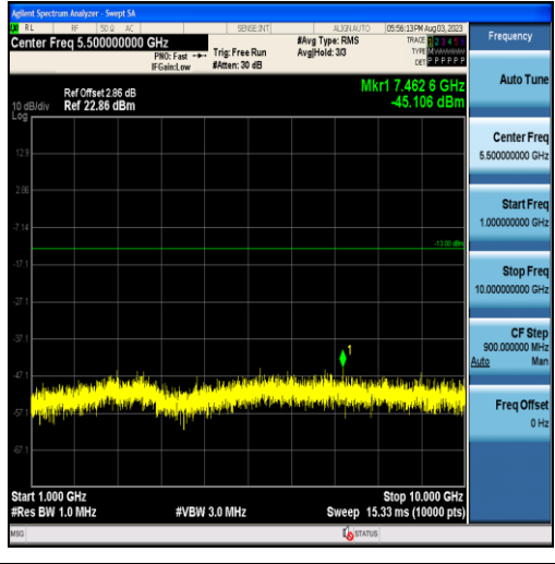
Band5-3MHz-QPSK-20415-15RB#0-Range2:1000~10000MHz
