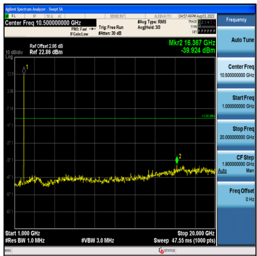
Band2-20MHz-QPSK-19100-100RB#0-Range2:1000~20000MHz
