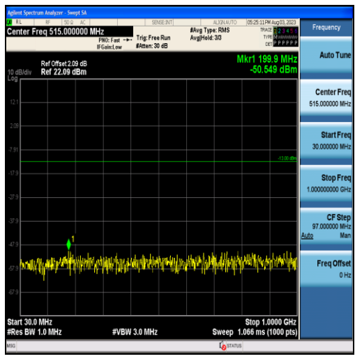
Band4-10MHz-QPSK-20000-50RB#0-Range1:30~1000MHz
