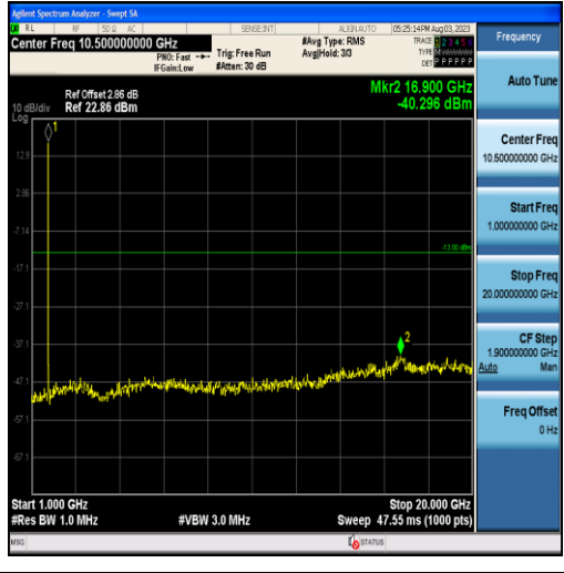
Band4-10MHz-QPSK-20000-50RB#0-Range2:1000~20000MHz
