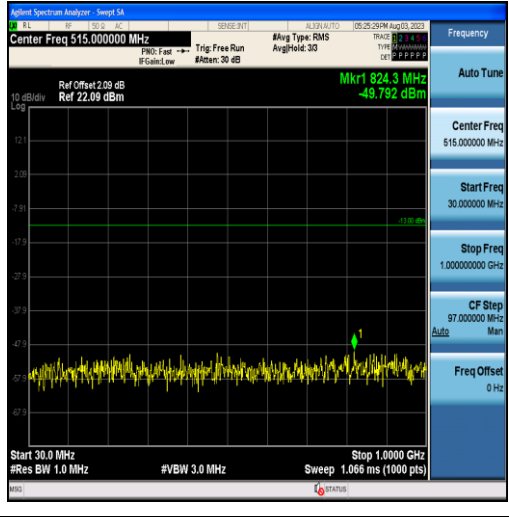
Band4-10MHz-QPSK-20175-50RB#0-Range1:30~1000MHz
