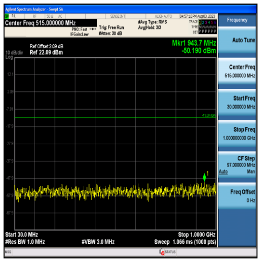
Band2-20MHz-QPSK-18700-100RB#0-Range1:30~1000MHz
