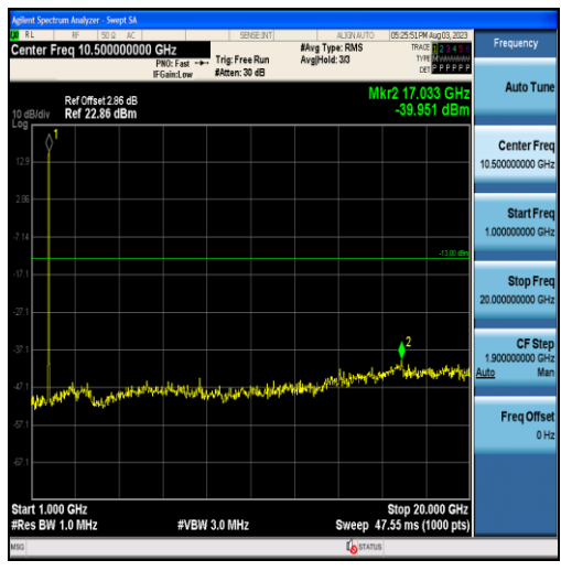
Band4-10MHz-QPSK-20350-50RB#0-Range2:1000~20000MHz
