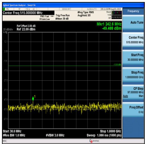
Band4-3MHz-QPSK-19965-15RB#0-Range1:30~1000MHz
