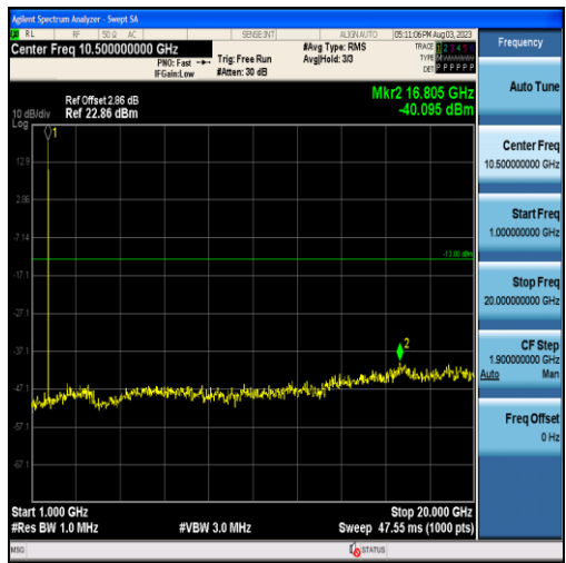
Band4-3MHz-QPSK-19965-15RB#0-Range2:1000~20000MHz
