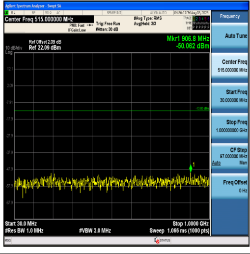
Band2-5MHz-QPSK-18900-25RB#0-Range1:30~1000MHz
