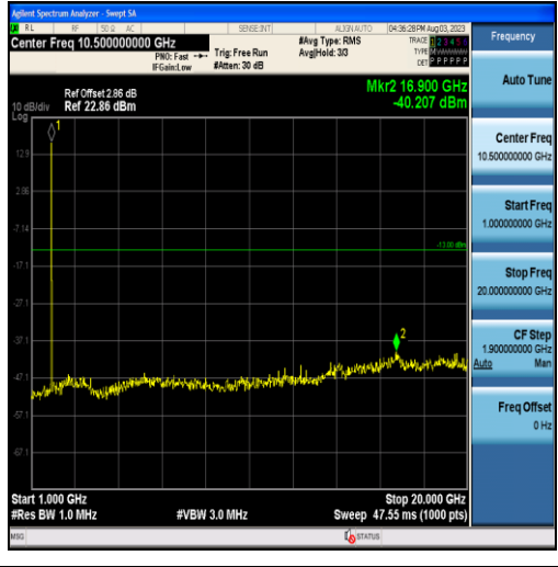
Band2-5MHz-16QAM-18900-25RB#0-Range2:1000~20000MHz
