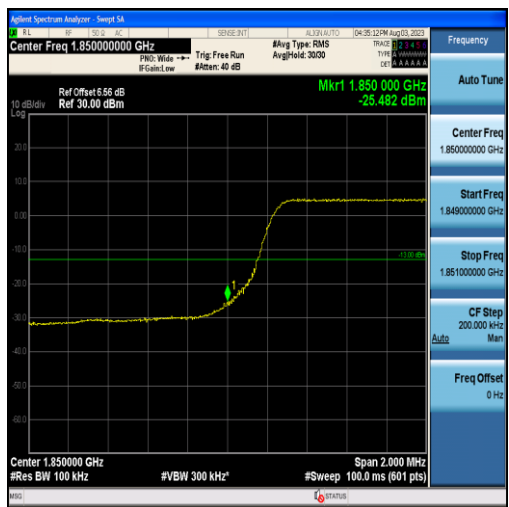
Band2-5MHz-QPSK-18625-25RB#0
