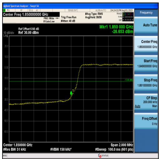
Band2-3MHz-16QAM-18615-15RB#0
