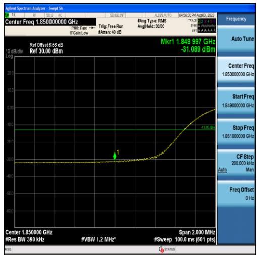
Band2-20MHz-16QAM-18700-100RB#0
