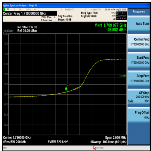
Band4-10MHz-QPSK-2000-50RB#0
