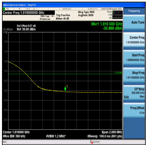
Band2-20MHz-16QAM-19100-100RB#0
