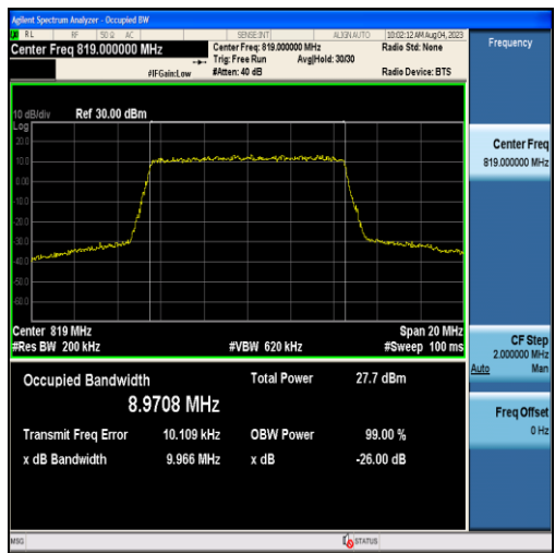
Band26-10MHz-QPSK-26740-50RB#0-8.9708
