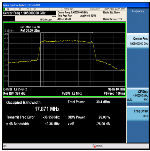
Band25-20MHz-QPSK-26590-100RB#0-17.871
