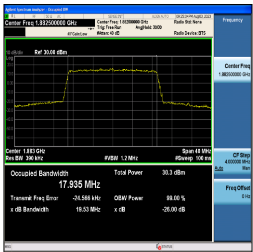
Band25-20MHz-QPSK-26365-100RB#0-17.935
