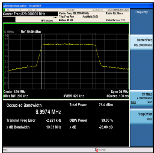
Band26-10MHz-QPSK-26840-50RB#0-8.9974
