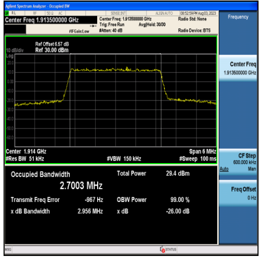
Band25-3MHz-QPSK-26675-15RB#0-2.7003
