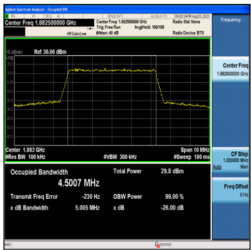
Band25-5MHz-QPSK-26365-25RB#0-4.5007
