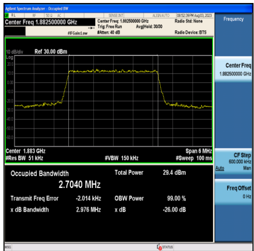
Band25-3MHz-QPSK-26365-15RB#0-2.7040
