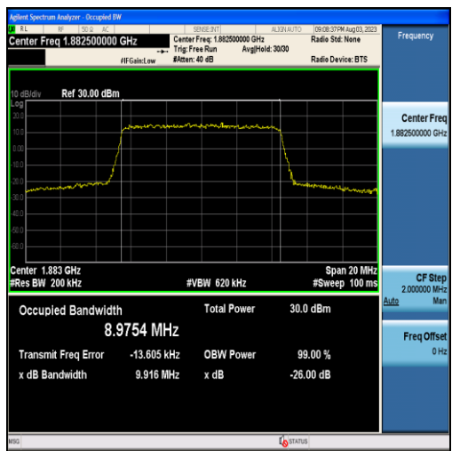
Band25-10MHz-QPSK-26365-50RB#0-8.9754
