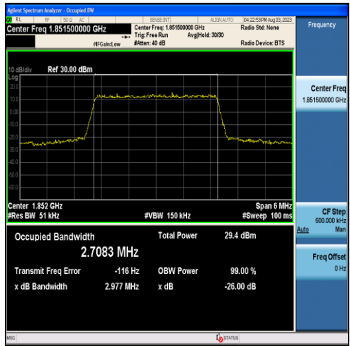
Band2-3MHz-QPSK-18615-15RB#0-2.7083
