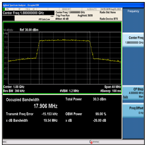
Band2-20MHz-QPSK-18900-100RB#0-17.906
