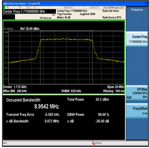
Band4-10MHz-QPSK-20000-50RB#0-8.9542
