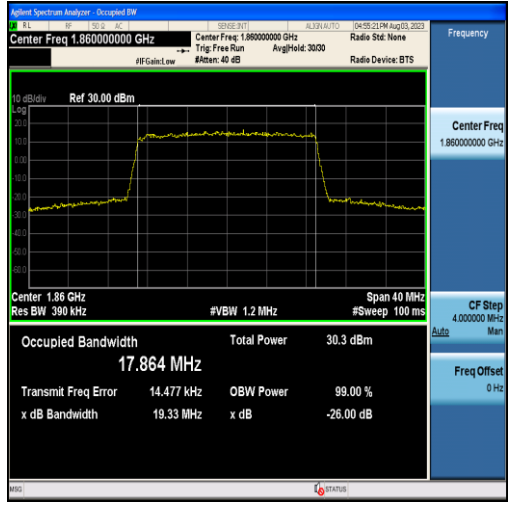
Band2-20MHz-QPSK-18700-100RB#0-17.864
