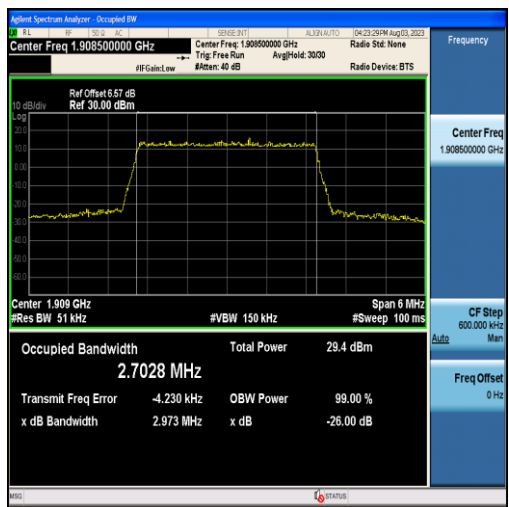
Band2-3MHz-QPSK-19185-15RB#0-2.7028
