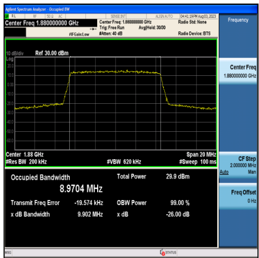
Band2-10MHz-QPSK-18900-50RB#0-8.9704
