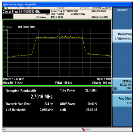
Band4-3MHz-QPSK-19965-15RB#0-2.7016
