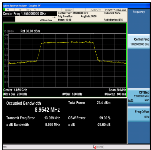
Band2-10MHz-16QAM-18650-50RB#0-8.9542
