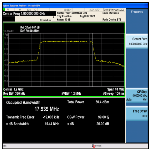
Band2-20MHz-QPSK-19100-100RB#0-17.939
