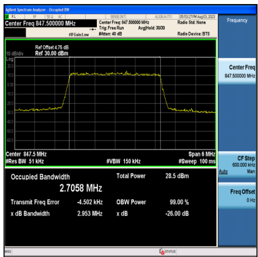
Band5-3MHz-QPSK-20635-15RB#0-2.7058
