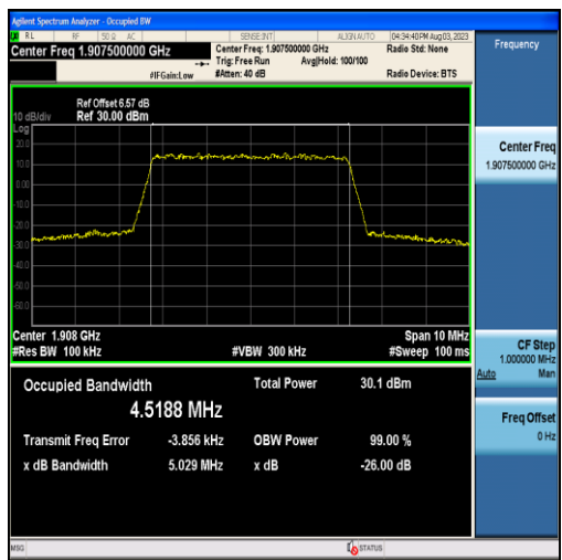
Band2-5MHz-QPSK-19175-25RB#0-4.5188
