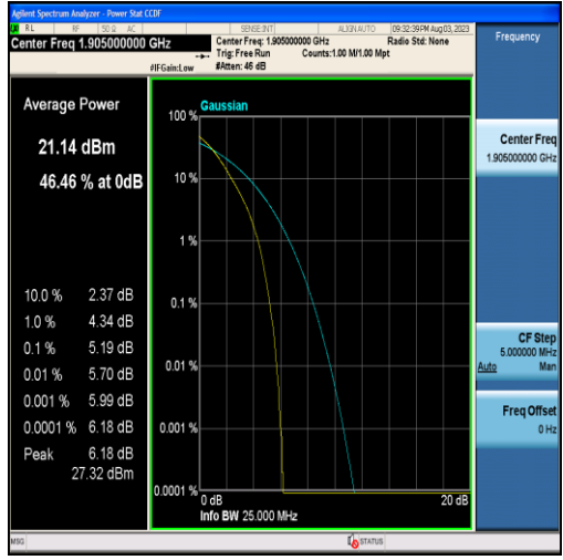
Band25-20MHz-QPSK-26590-100RB#0
