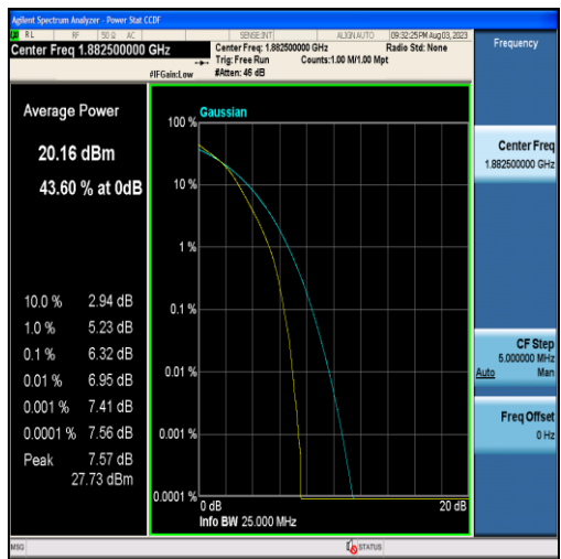
Band25-20MHz-16QAM-26365-100RB#0
