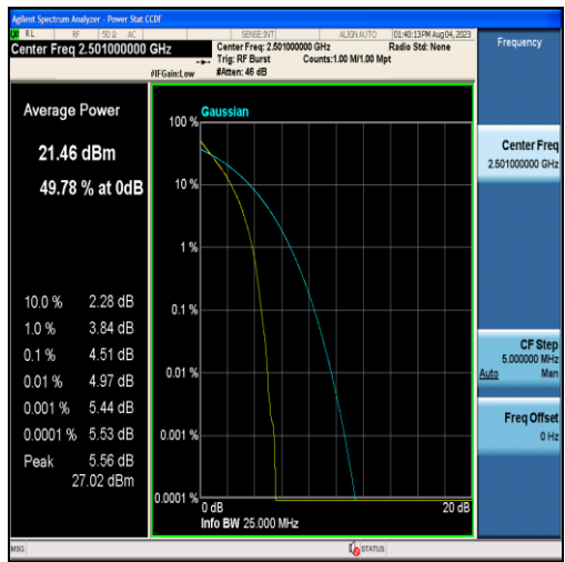
Band41-10MHz-QPSK-39700-50RB#0
