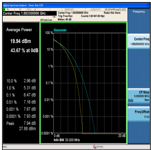
Band25-10MHz-16QAM-26365-50RB#0
