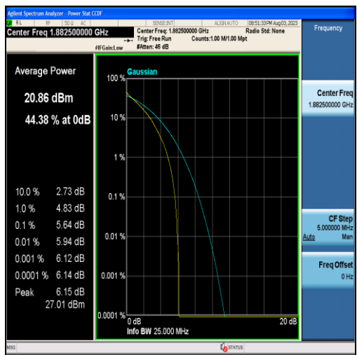
Band25-1.4MHz-QPSK-26365-6RB#0
