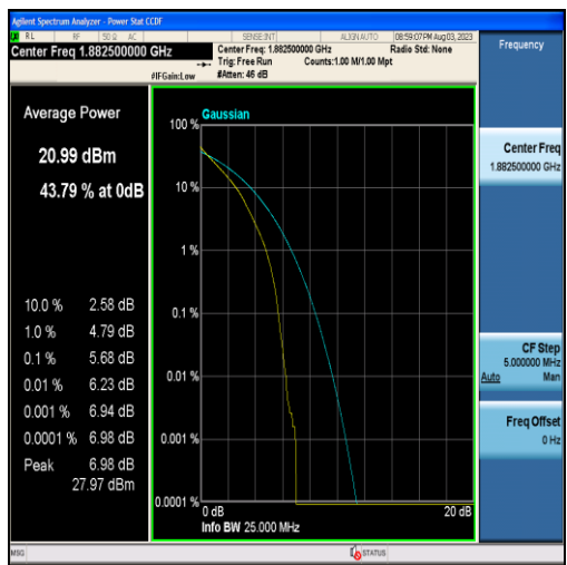
Band25-3MHz-QPSK-26365-15RB#0
