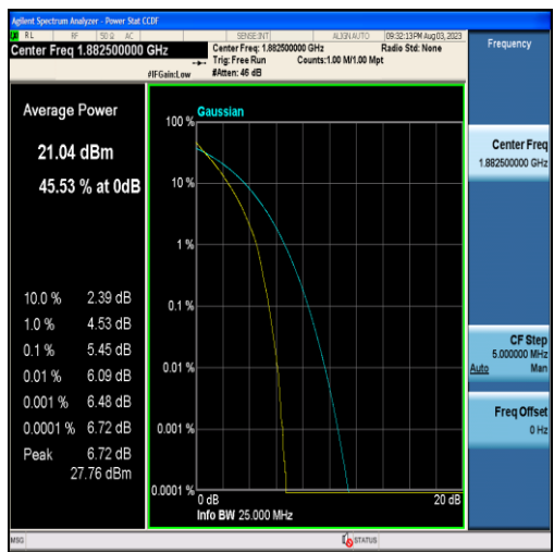
Band25-20MHz-QPSK-26365-100RB#0
