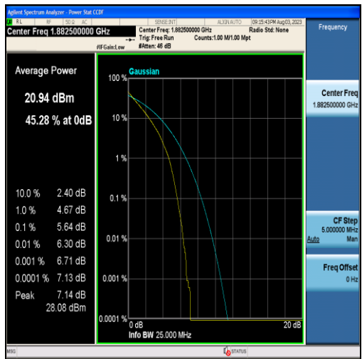
Band25-10MHz-QPSK-26365-50RB#0
