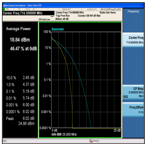
Band12-3MHz-QPSK-23165-15RB#0
