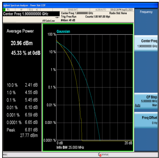
Band2-20MHz-QPSK-19100-100RB#0
