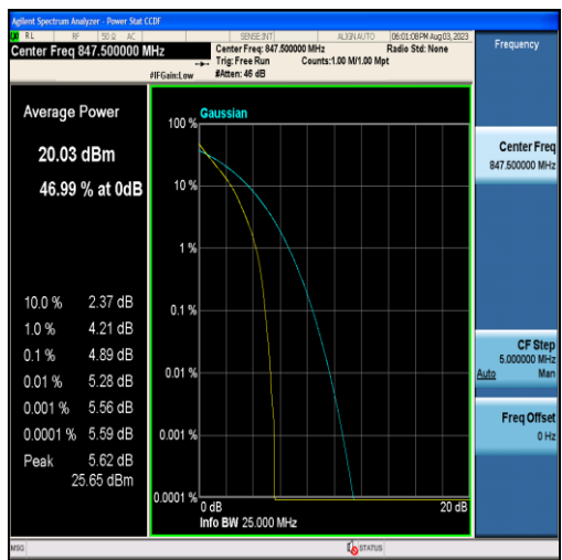
Band5-3MHz-QPSK-20635-15RB#0
