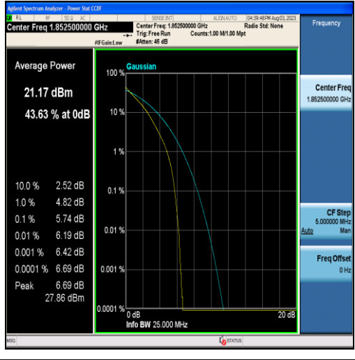
Band2-5MHz-QPSK-18625-25RB#0
