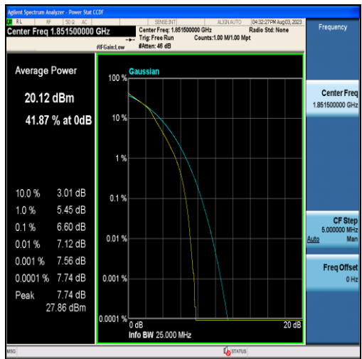
Band2-3MHz-16QAM-18615-15RB#0
