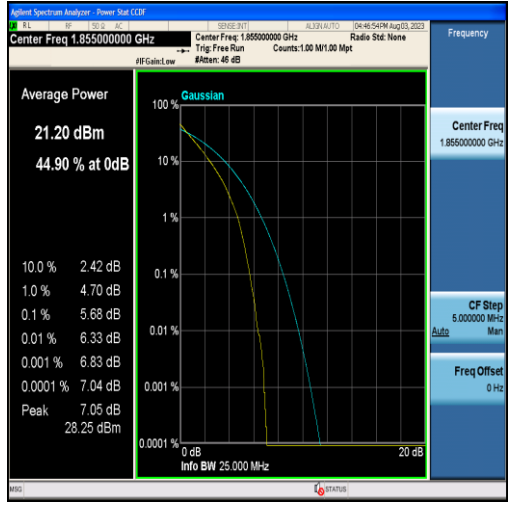
Band2-10MHz-QPSK-18650-50RB#0
