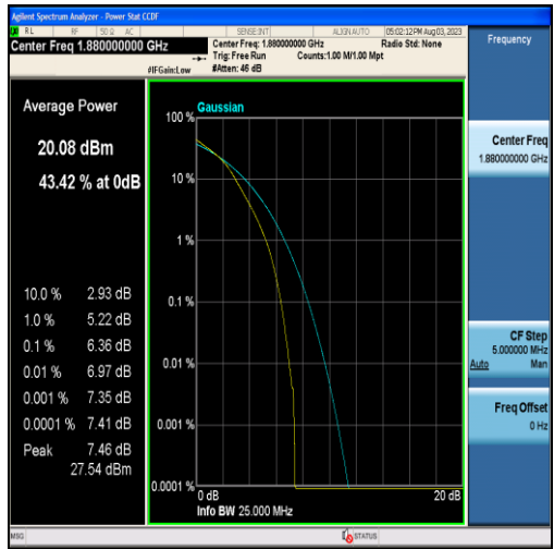
Band2-20MHz-16QAM-18900-100RB#0
