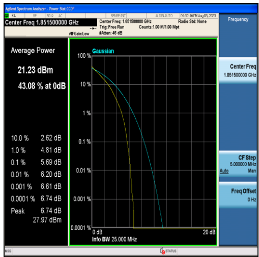
Band2-3MHz-QPSK-18615-15RB#0
