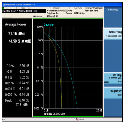
Band2-3MHz-QPSK-19185-15RB#0
