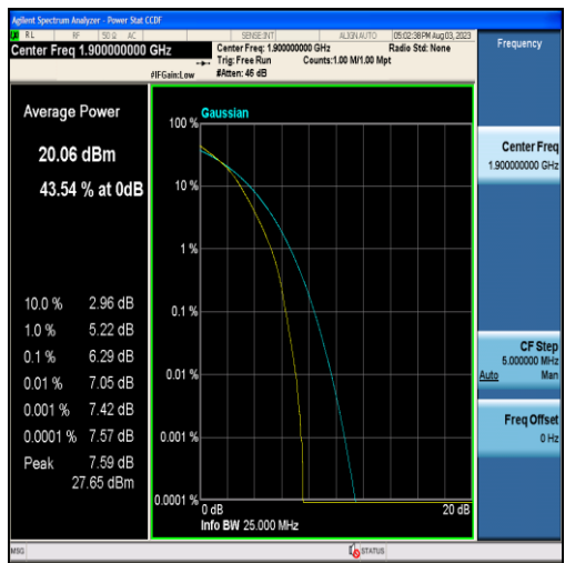
Band2-20MHz-16QAM-19100-100RB#0
