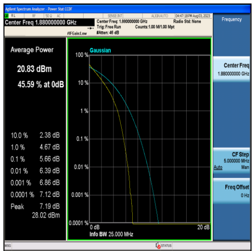
Band2-10MHz-QPSK-18900-50RB#0
