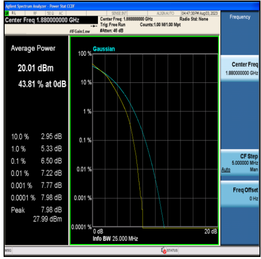
Band2-10MHz-16QAM-18900-50RB#0
