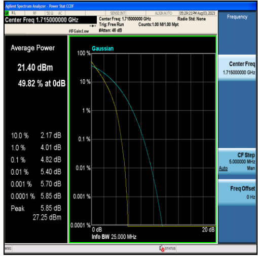
Band4-10MHz-QPSK-20000-50RB#0
