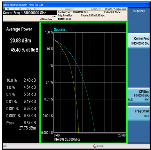
Band2-20MHz-QPSK-18900-100RB#0
