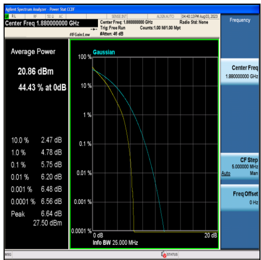
Band2-5MHz-QPSK-18900-25RB#0
