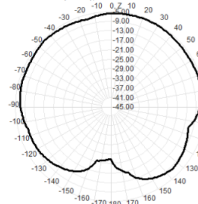
825.0MHz Total(E2-YZ), Max=-5.54dBi
