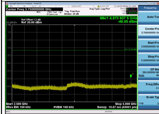
802.11b,2437MHz,Ant0,Plot 4,2500MHz~5000MHz
