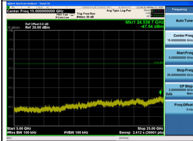
802.11n(HT20),2462MHz,Ant0,Plot 5,5000MHz~25000MHz
