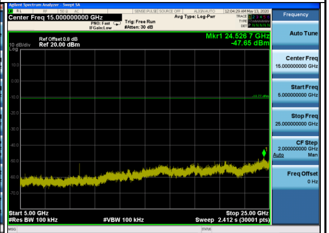
802.11b,2437MHz,Ant0,Plot 5,5000MHz~25000MHz
