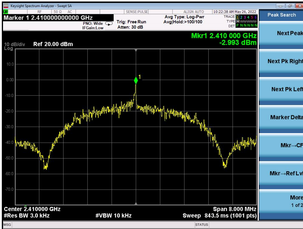
GFSK-2410MHz
