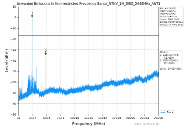
30MHz-25GHz CH19
