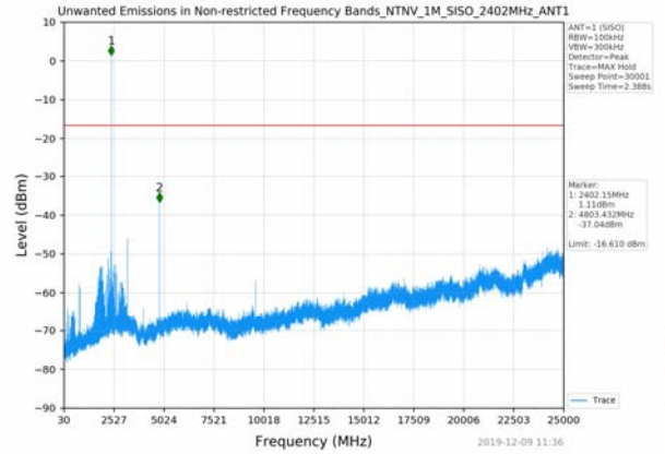
30MHz-25GHz CH00
