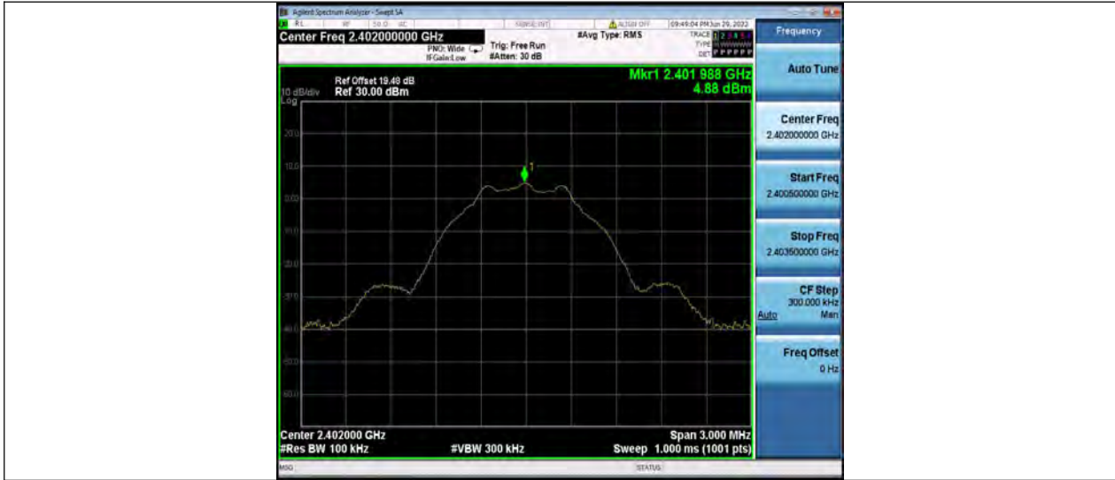
BLE 1M Ant1 2402 0~Reference
