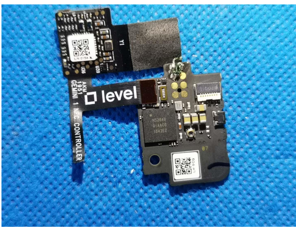
(2) EUT Photo
