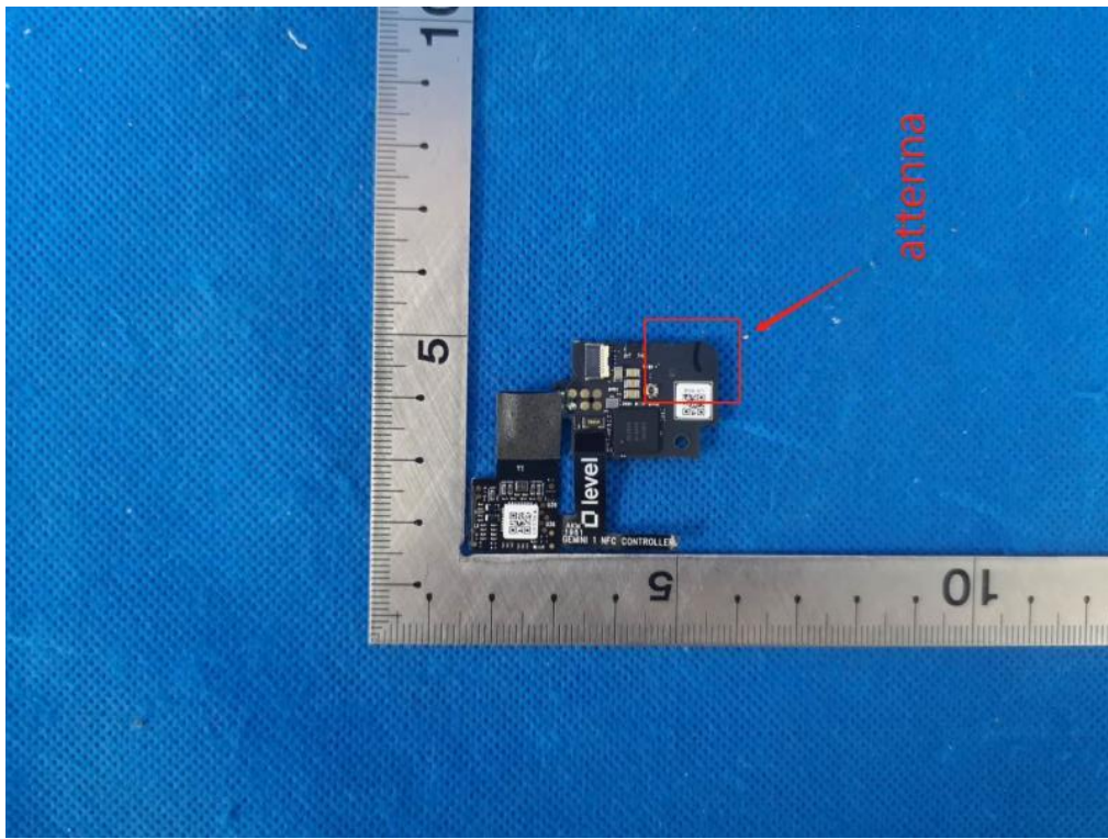
(3) EUT Photo
