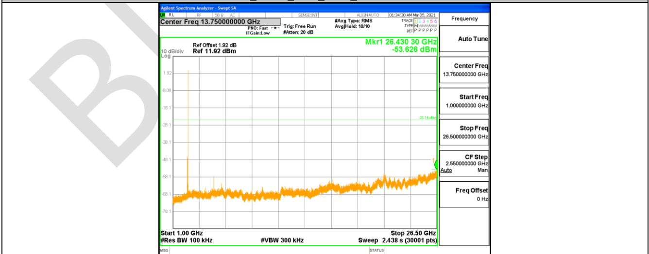
BLE BT4.0_Ant1_2480_1000~26500
