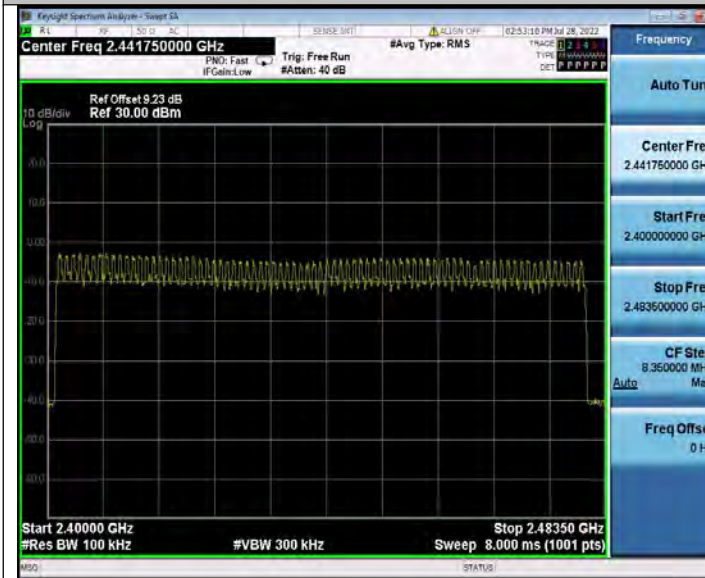
8DPSK
