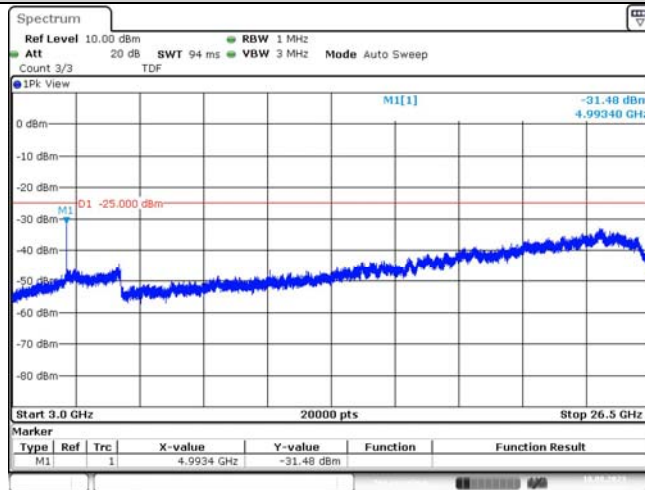
Band41-5MHz-QPSK-39675-1RB#0-Range3:3000~26500MHz
