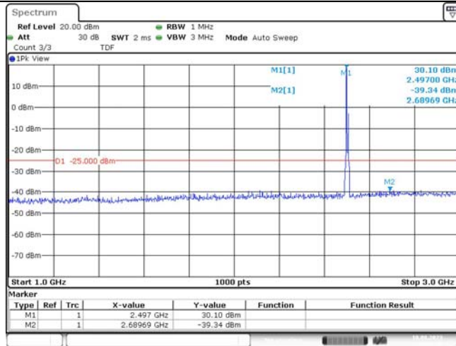
Band41-5MHz-QPSK-39675-1RB#0-Range2:1000~3000MHz
