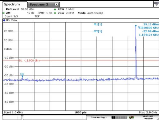
Band25-1.4MHz-QPSK-26047-1RB#0-Range2:1000~2000MHz
