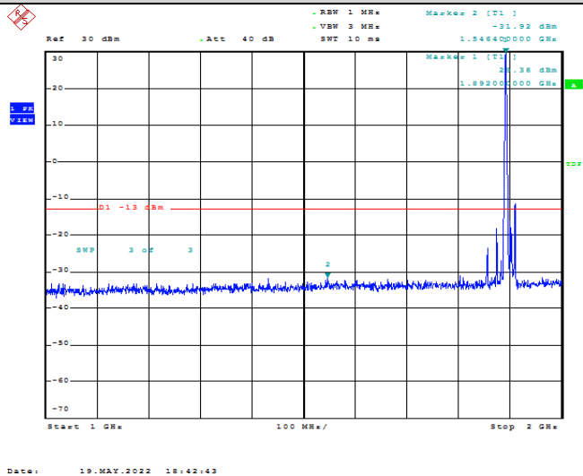
Band2-20MHz-16QAM-19100-1RB#0-Range2:1000~2000MHz
