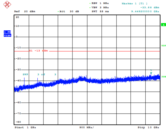
Band26-1.4MHz-QPSK-26697-1RB#0-Range2:1000~10000MHz
